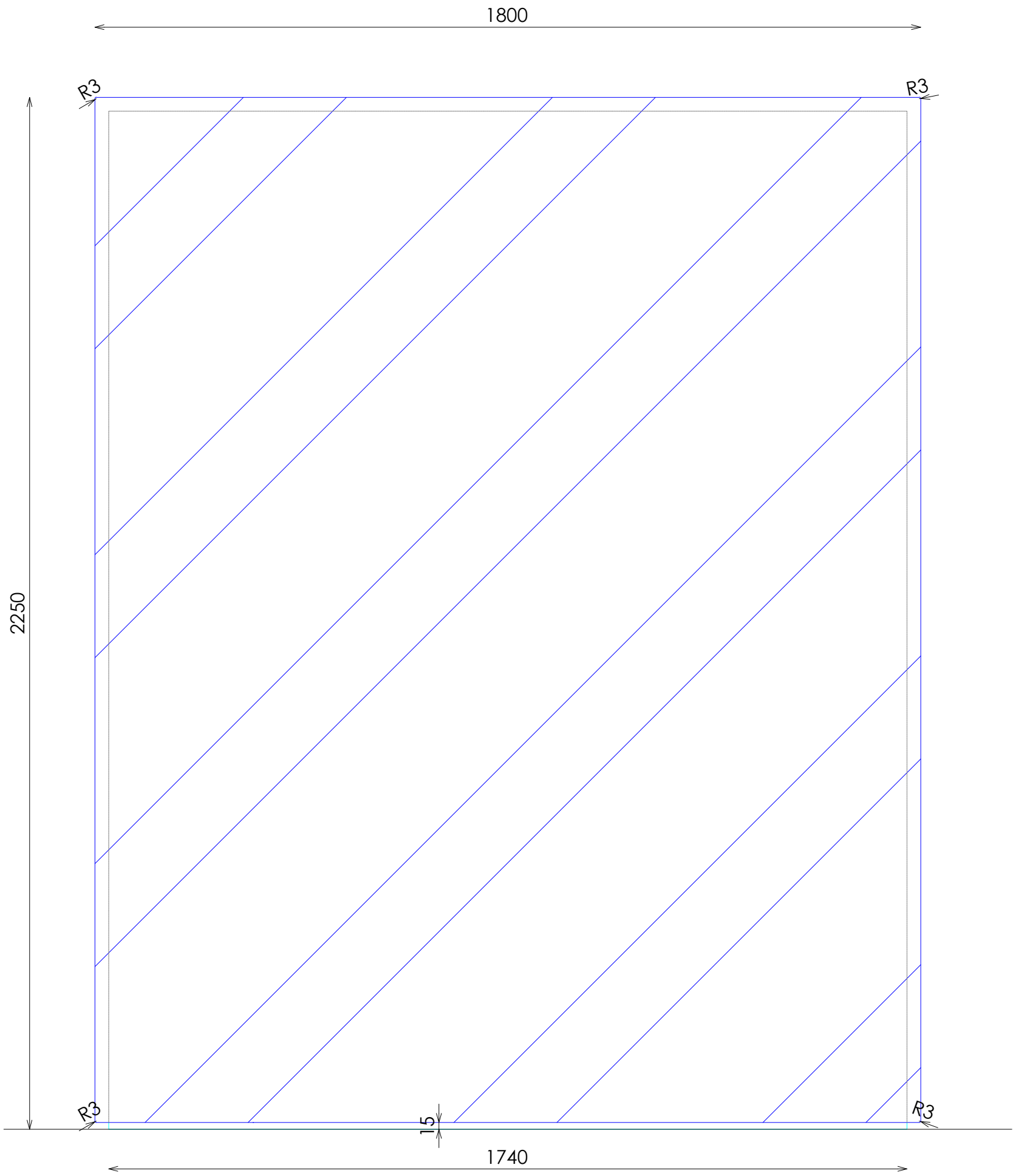
ALZADO CONJUNTO
