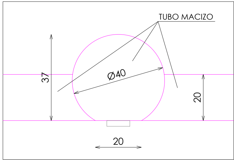
DETALLE D
