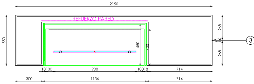
PLANTA
