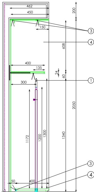
SECCIÓN
