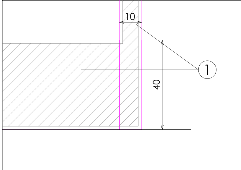
DETALLE C
