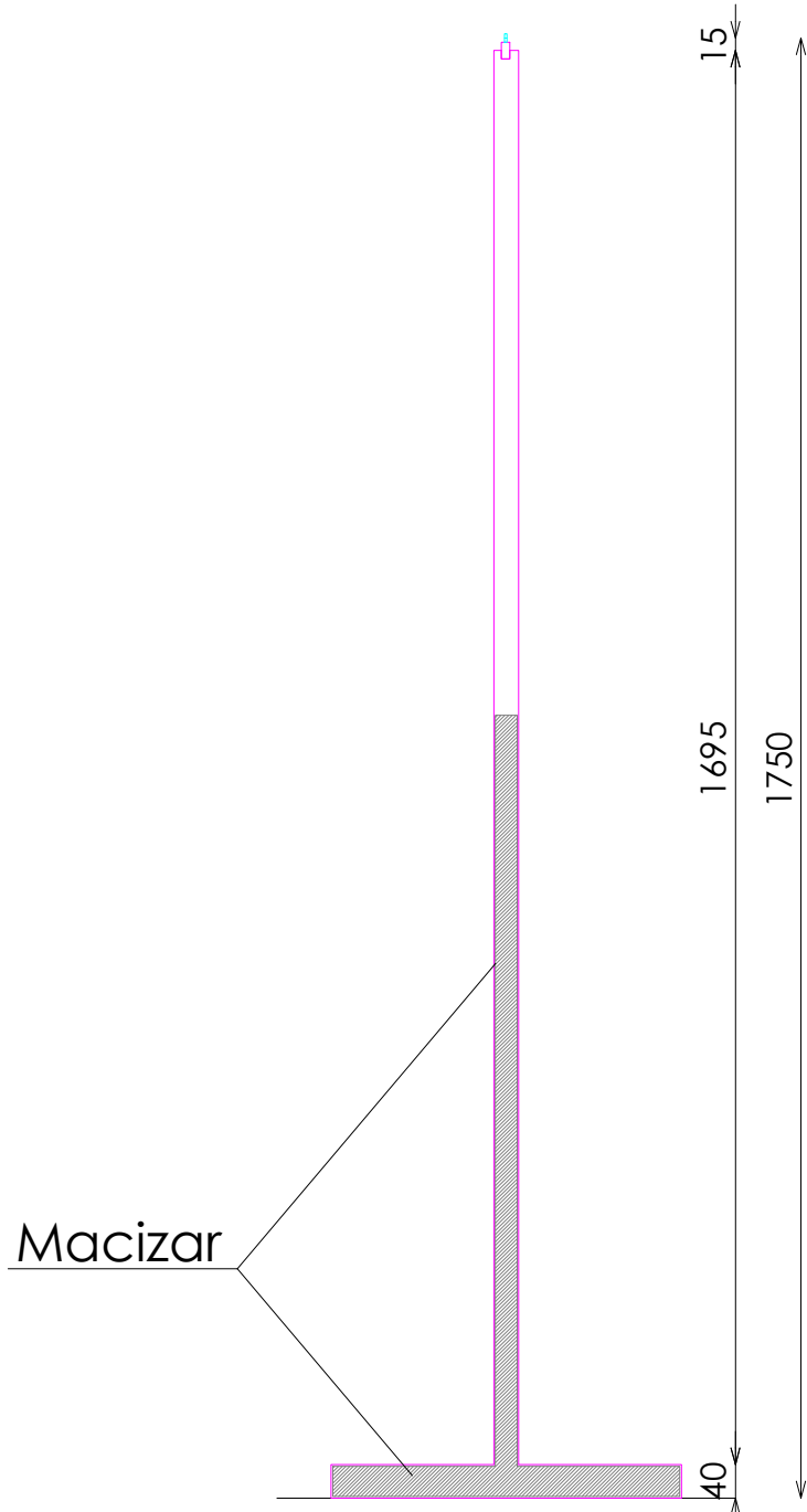
SECCIÓN
