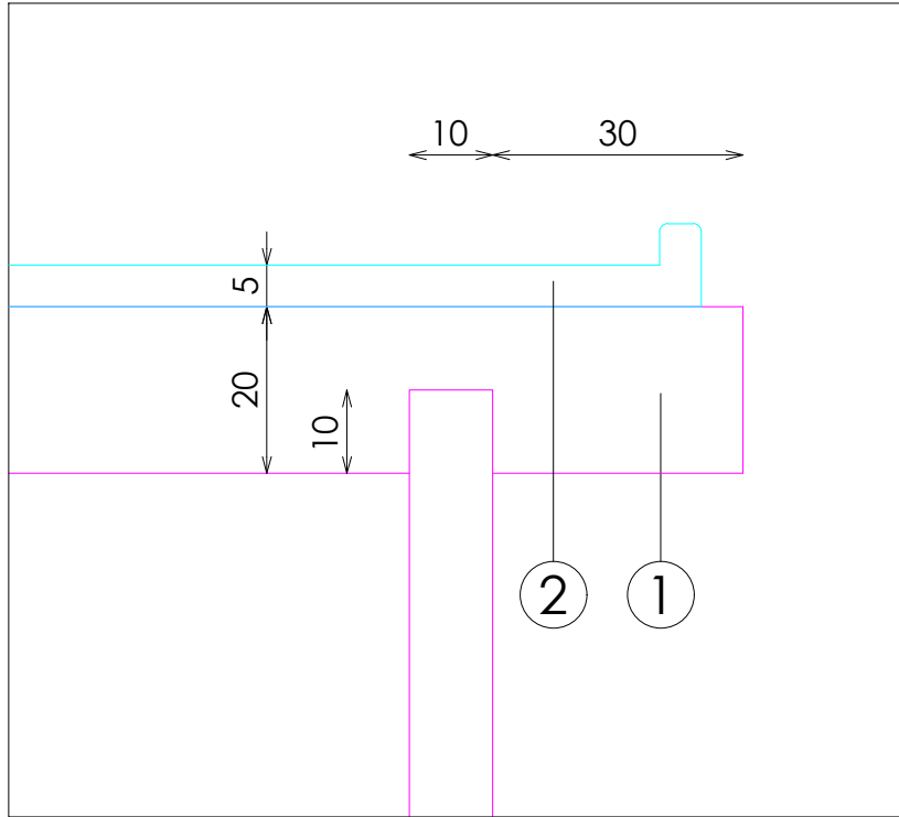
DETALLE C
