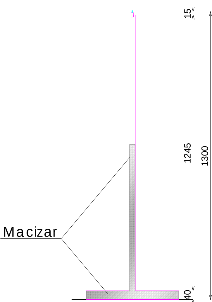
SECCIÓN
