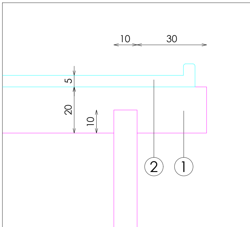
DETALLE B
