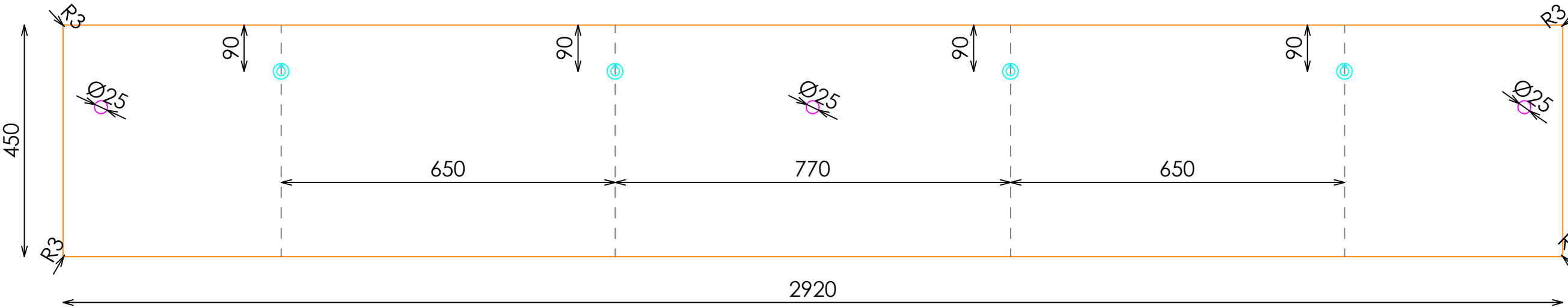
PLANTA TARIMA (POSICIONES COLGADORES AUXILIARES)
