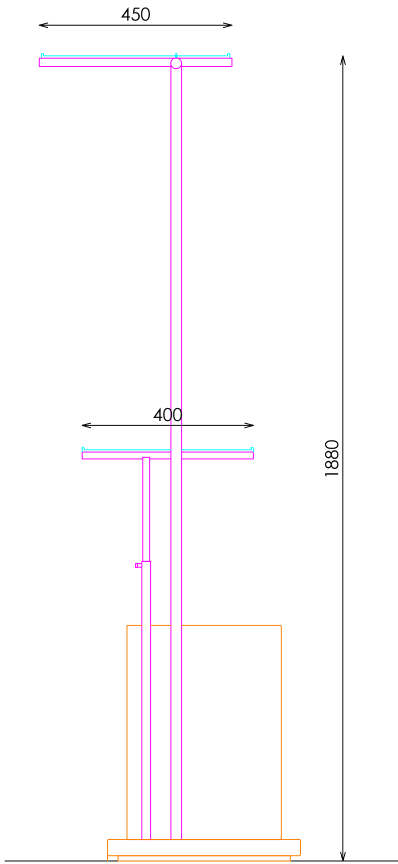
ALZADO LATERAL
