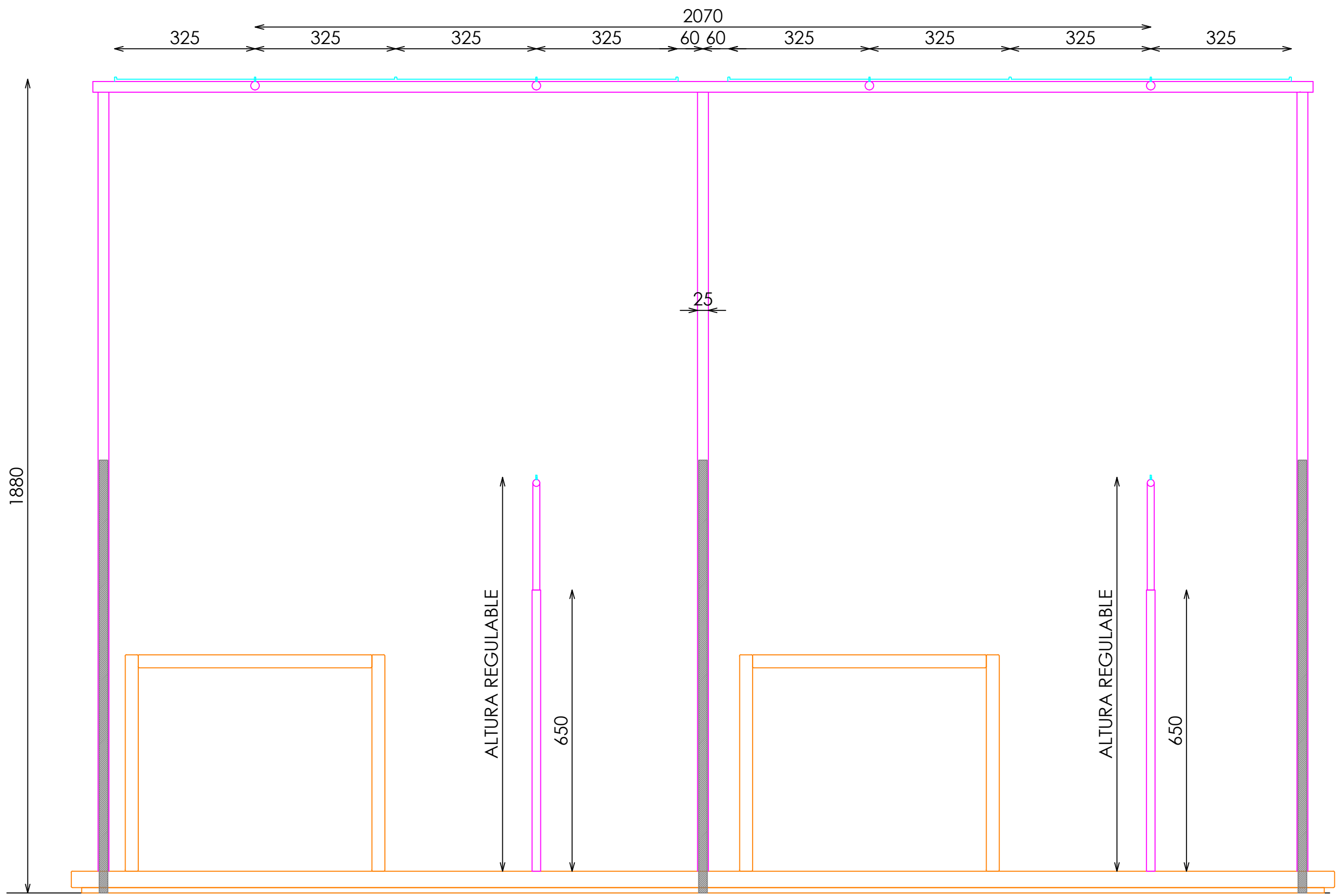
ALZADO FRONTAL
