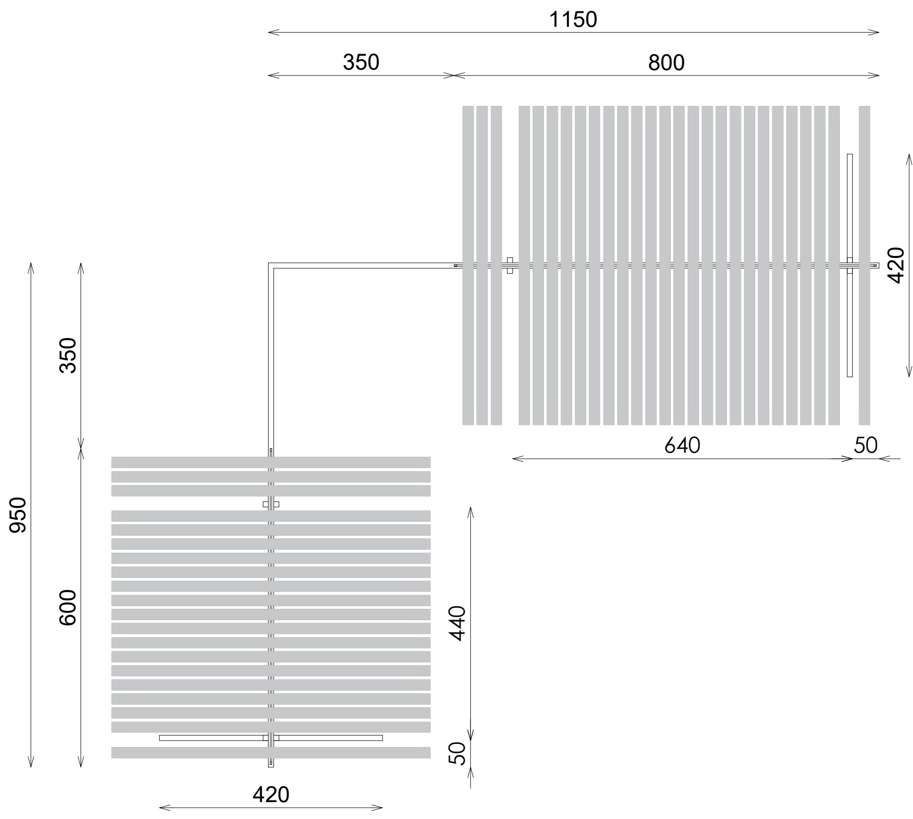
PLANTA
