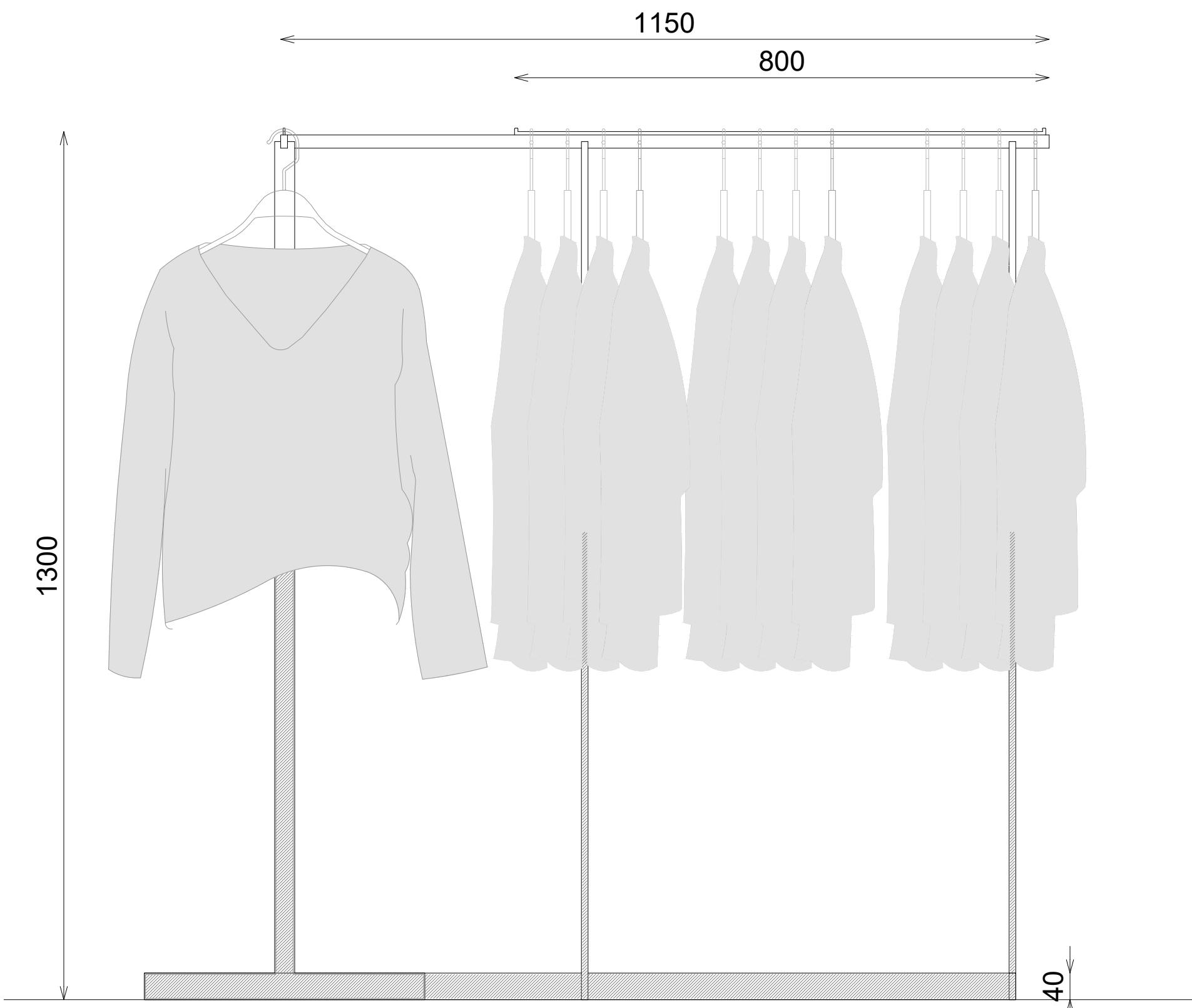
ALZADO FRONTAL
