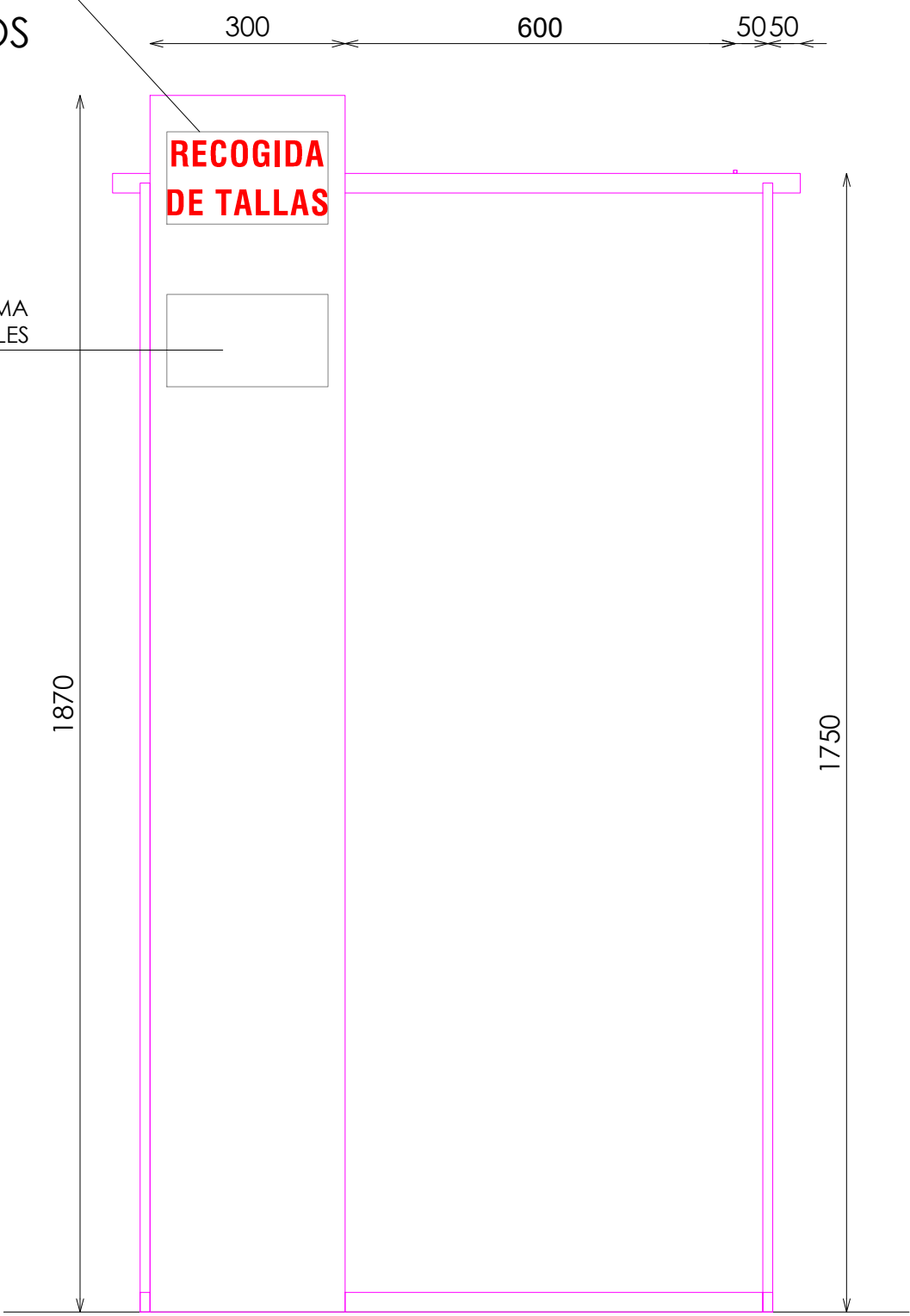
ALZADO FRONTAL
