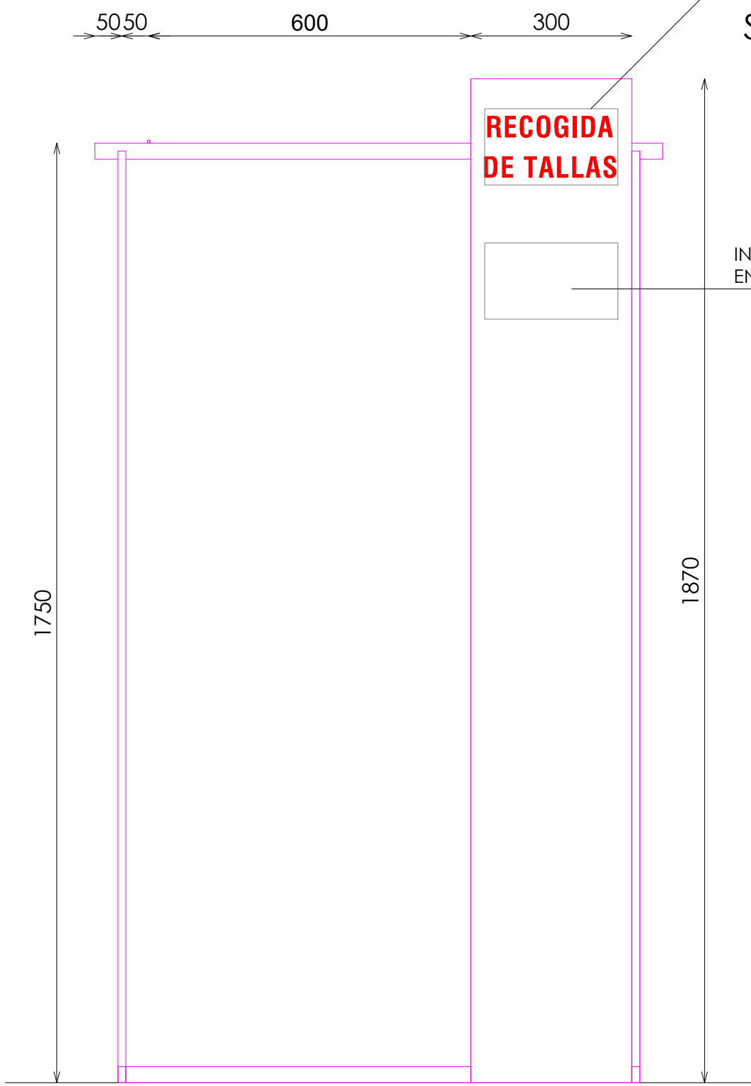
ALZADO POSTERIOR
