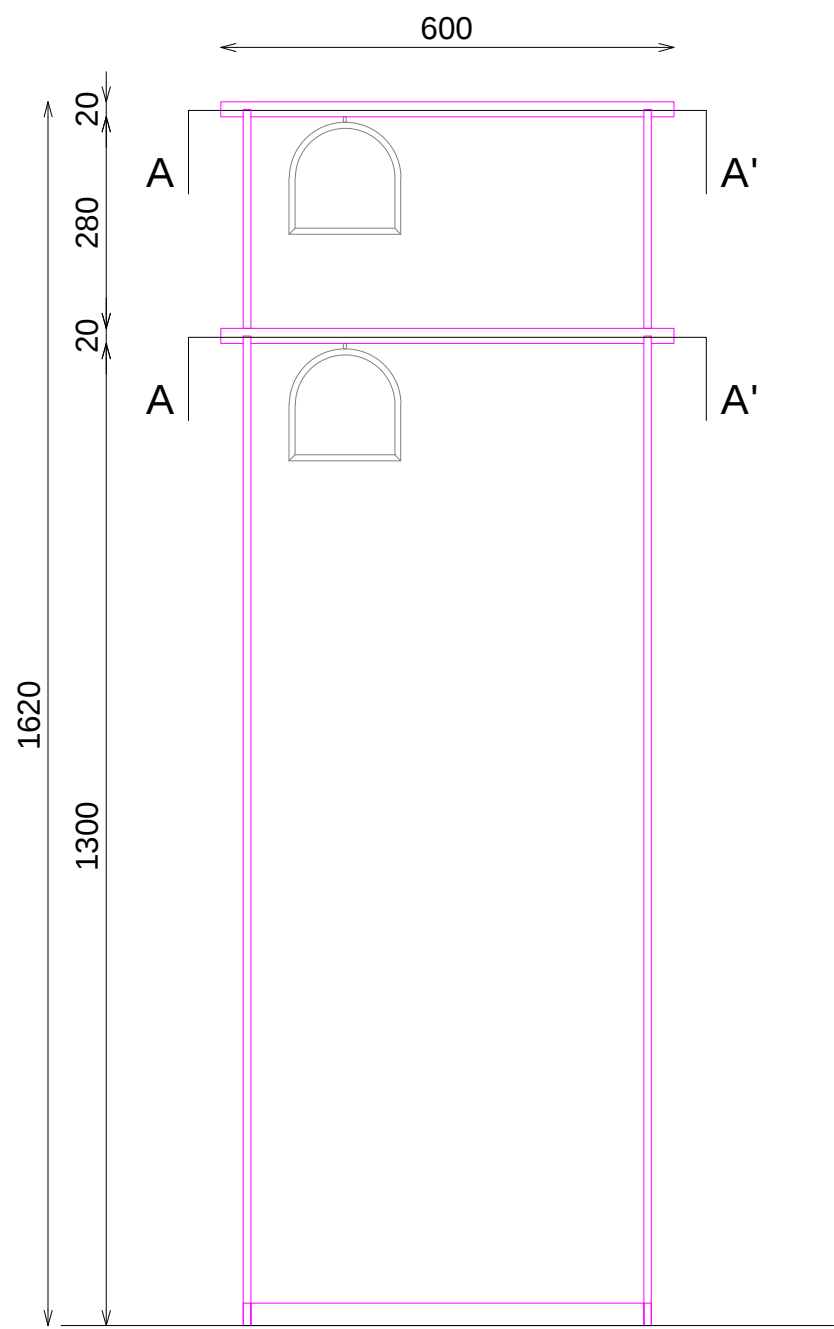
ALZADO
