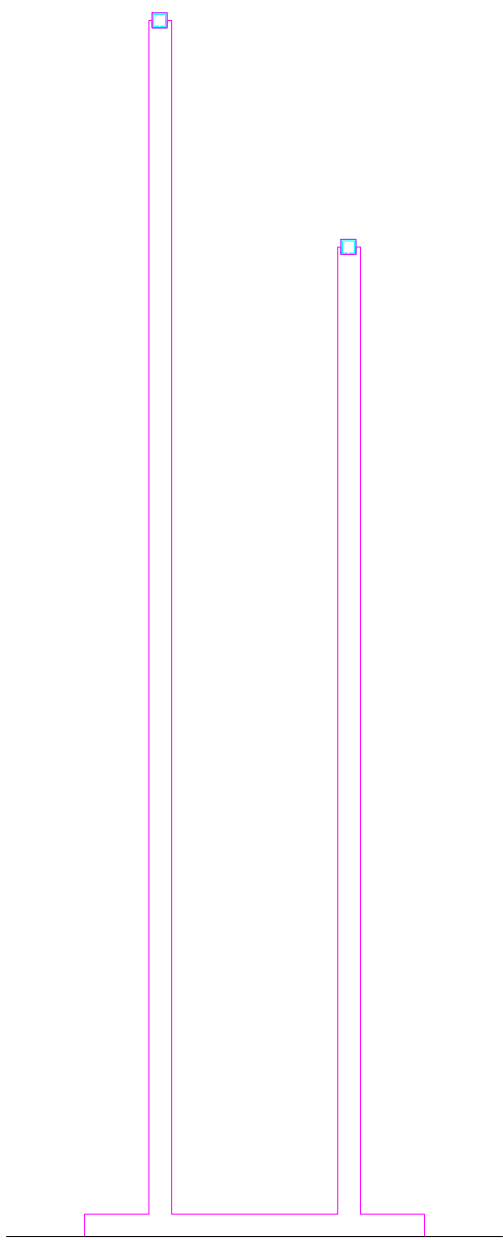
SECCIÓN
