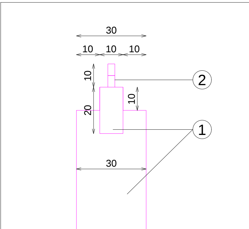
DETALLE A
