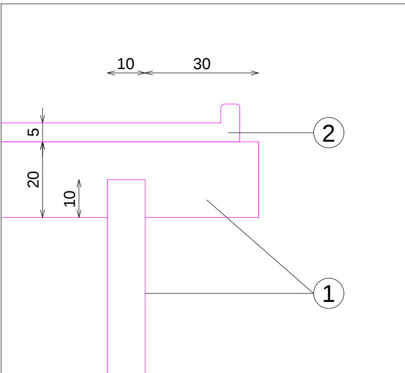
DETALLE B
