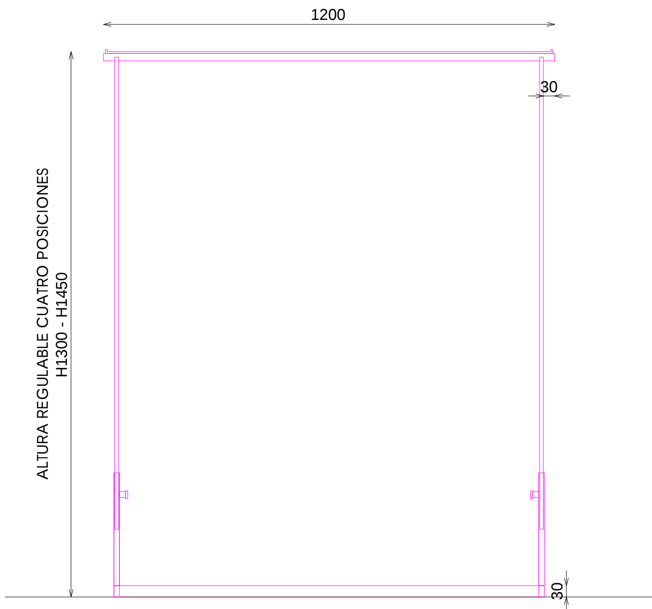
ALZADO
