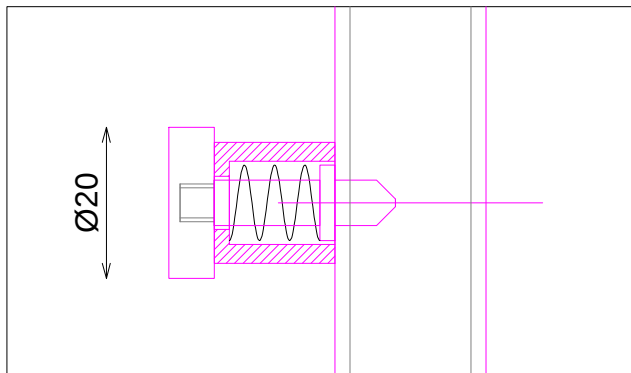
DETALLE SISTEMA ANCLAJE
