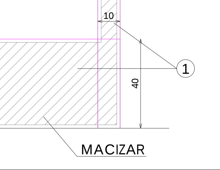
DETALLE C
