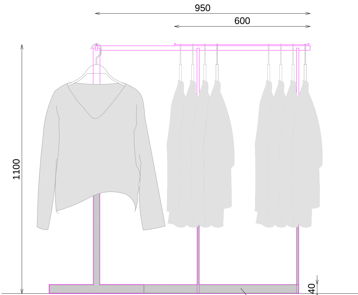
ALZADO LATERAL
