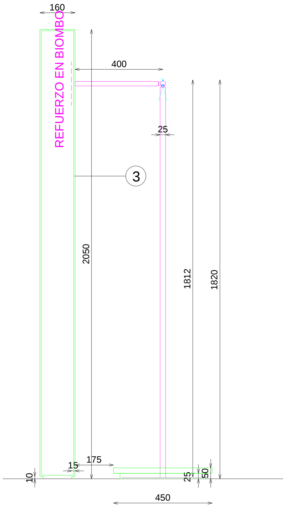
PERFIL
