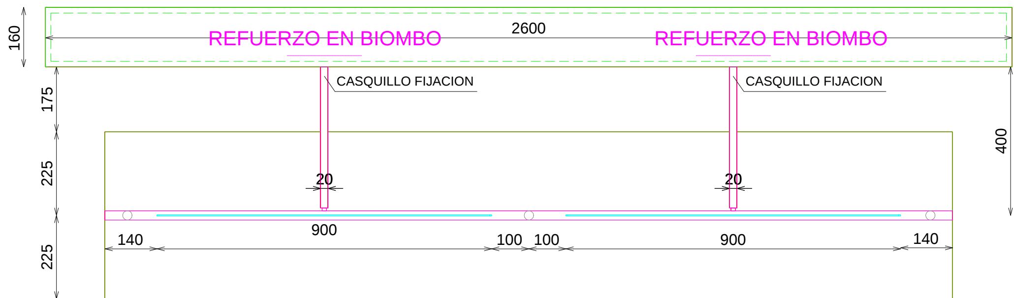
PLANTA
