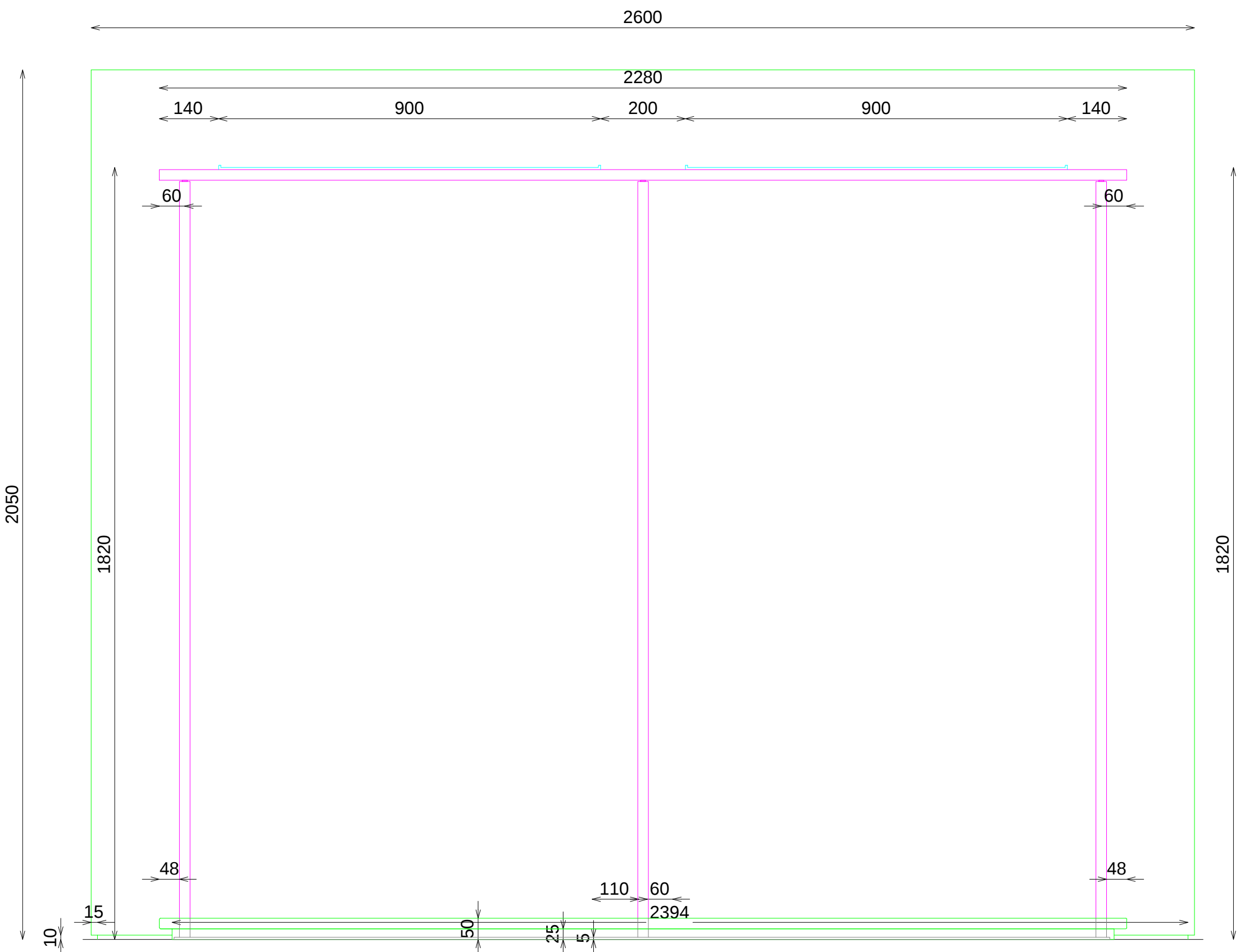
ALZADO
