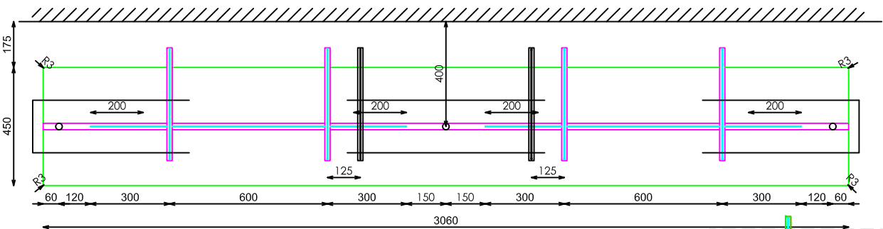
PLANTA
