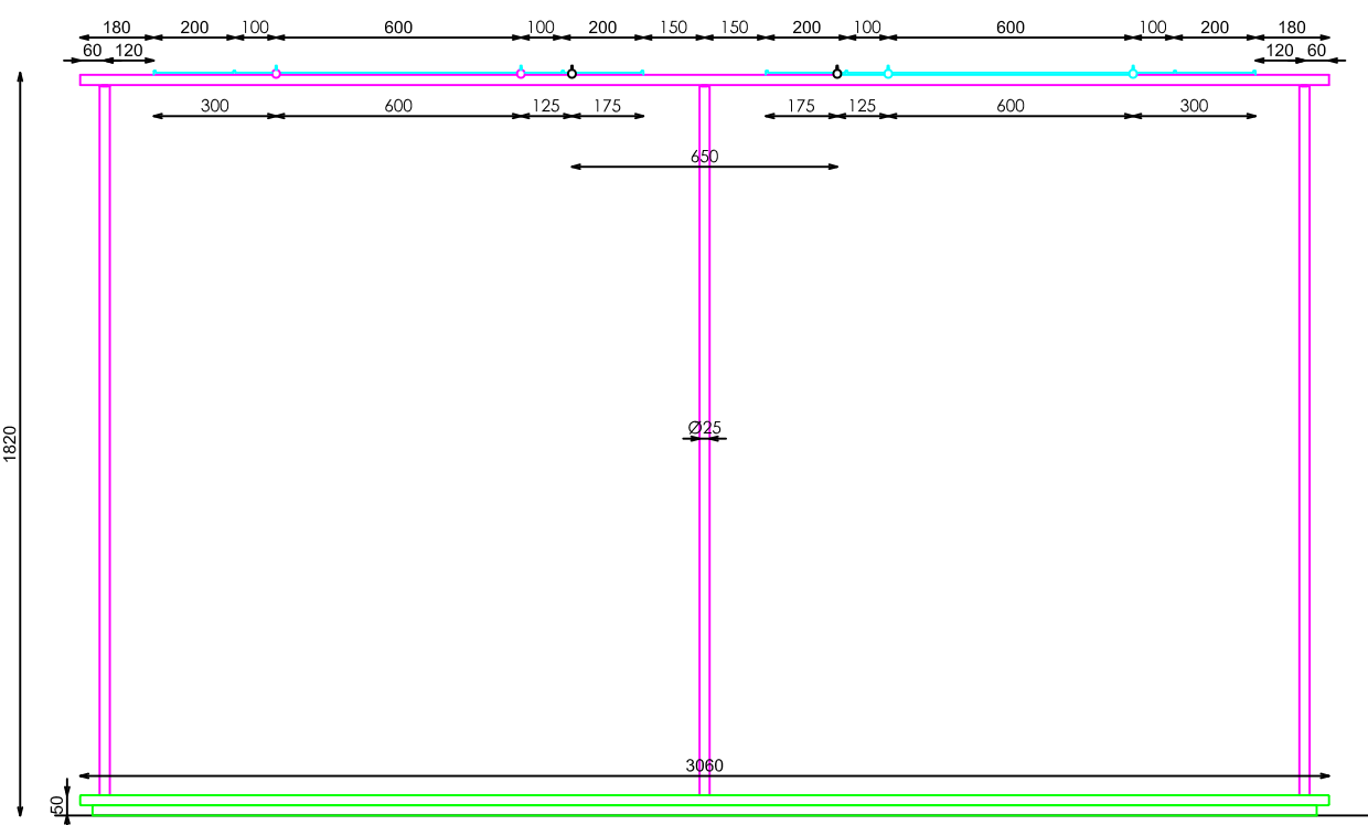
ALZADO FRONTAL
