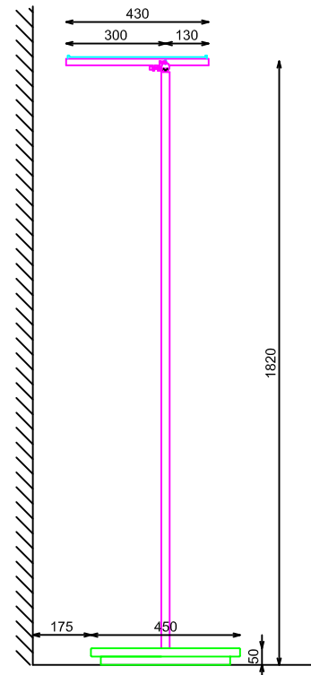
SECCIÓN
