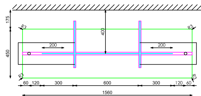
PLANTA
