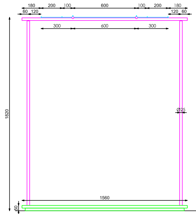
ALZADO FRONTAL
