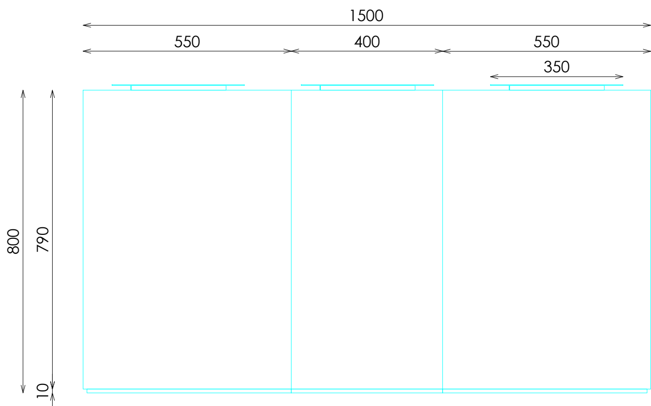
ALZADO DELANTERO
