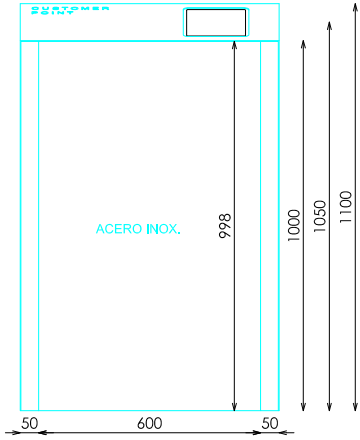
ALZADO
