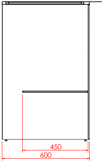
剖面 AH-AH
