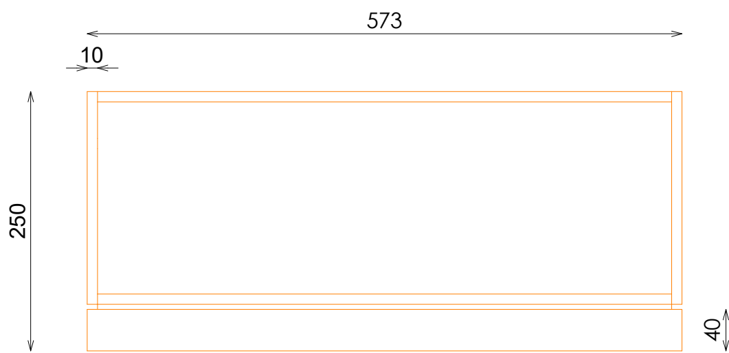
ALZADO
