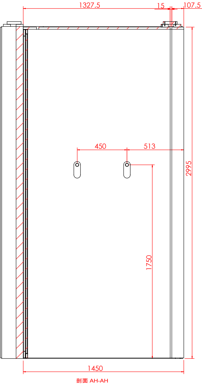
剖面 AH-AH
