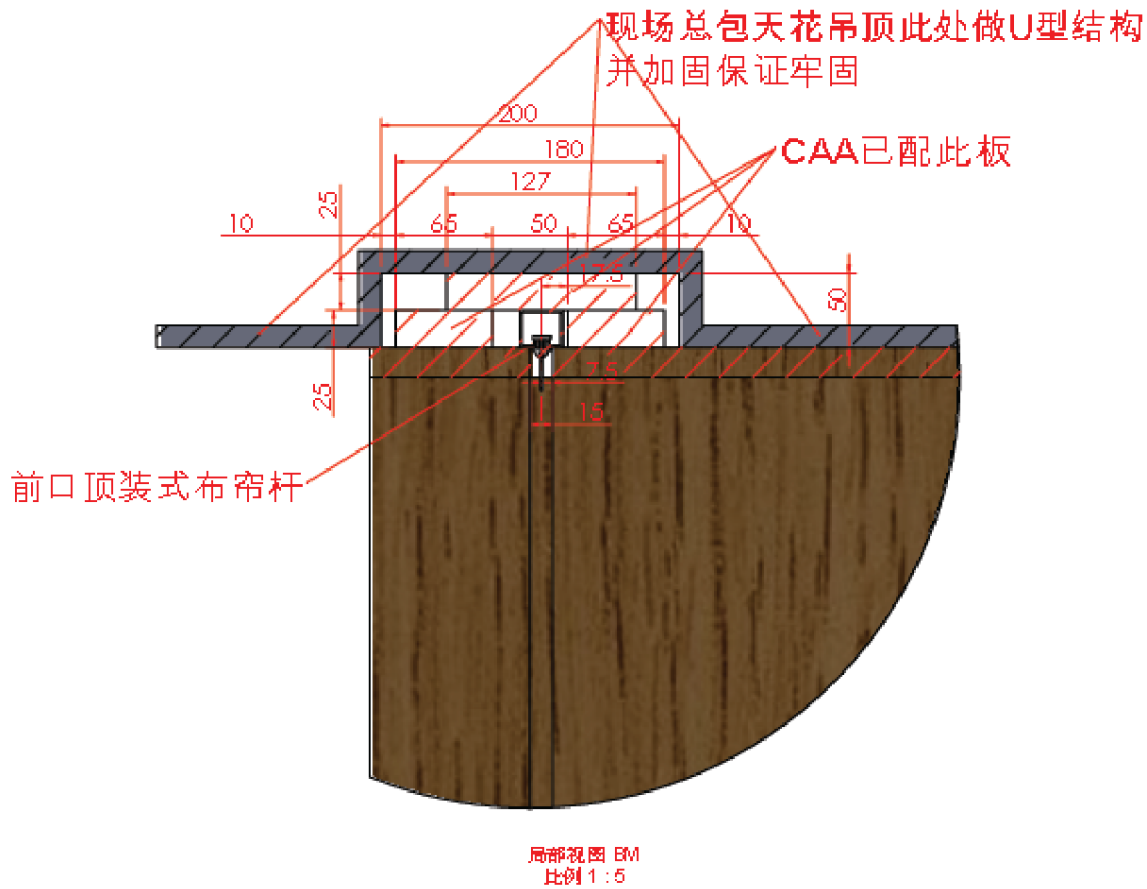
顶上布帘杆天花顶要求及 安装示意图
