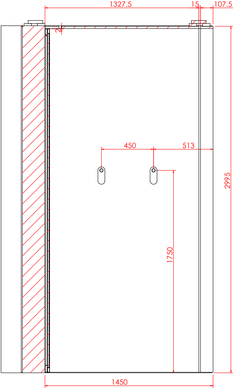
剖面 AI-AI
