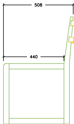
PERFIL SIDE ELEVATION
