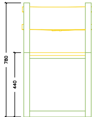
ALZADO ELEVATION
