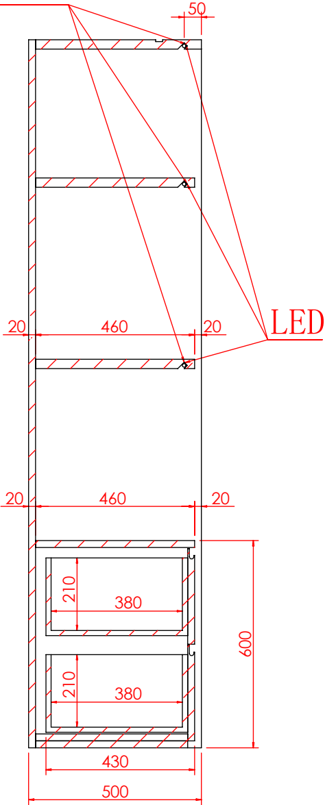
剖面 AG-AG
