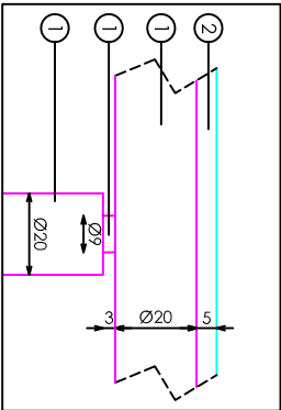
DETALLE A
