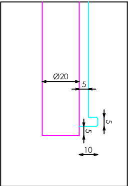
DETALLE B
