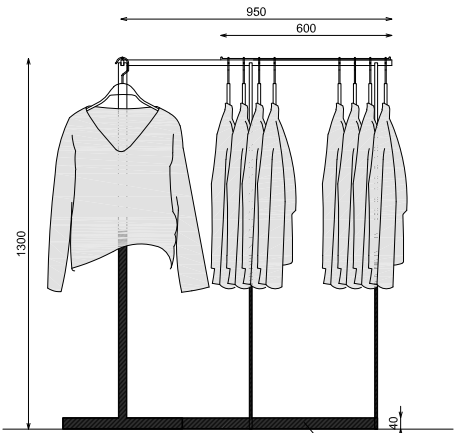
ALZADO LATERAL
