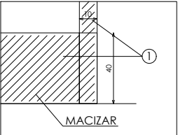
DETALLE C
