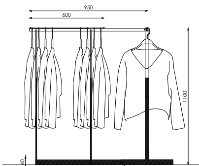
ALZADO LATERAL
