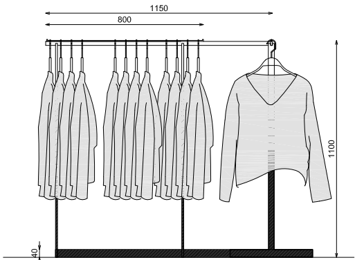
ALZADO FRONTAL
