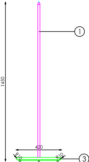
PERFIL
