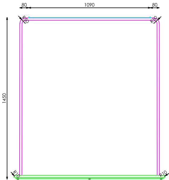
ALZADO
