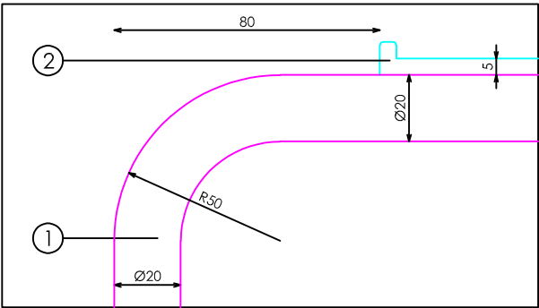
DETALLE A
