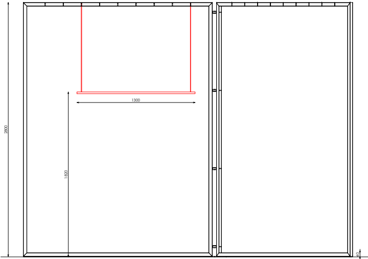
ALZADO
