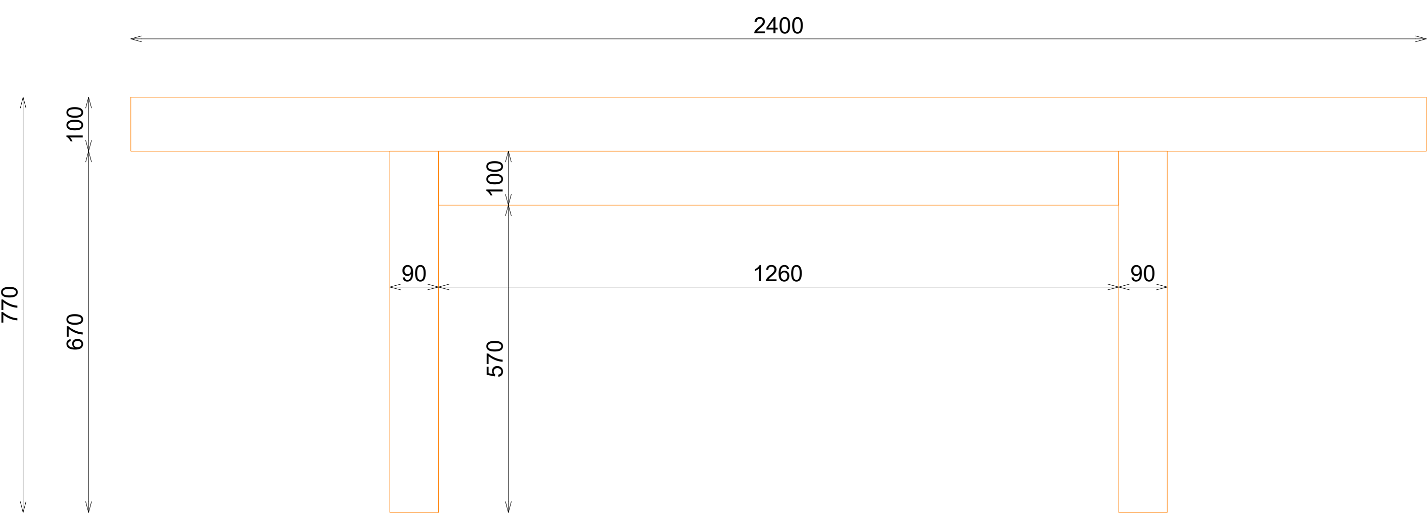
ALZADO FRONTAL
