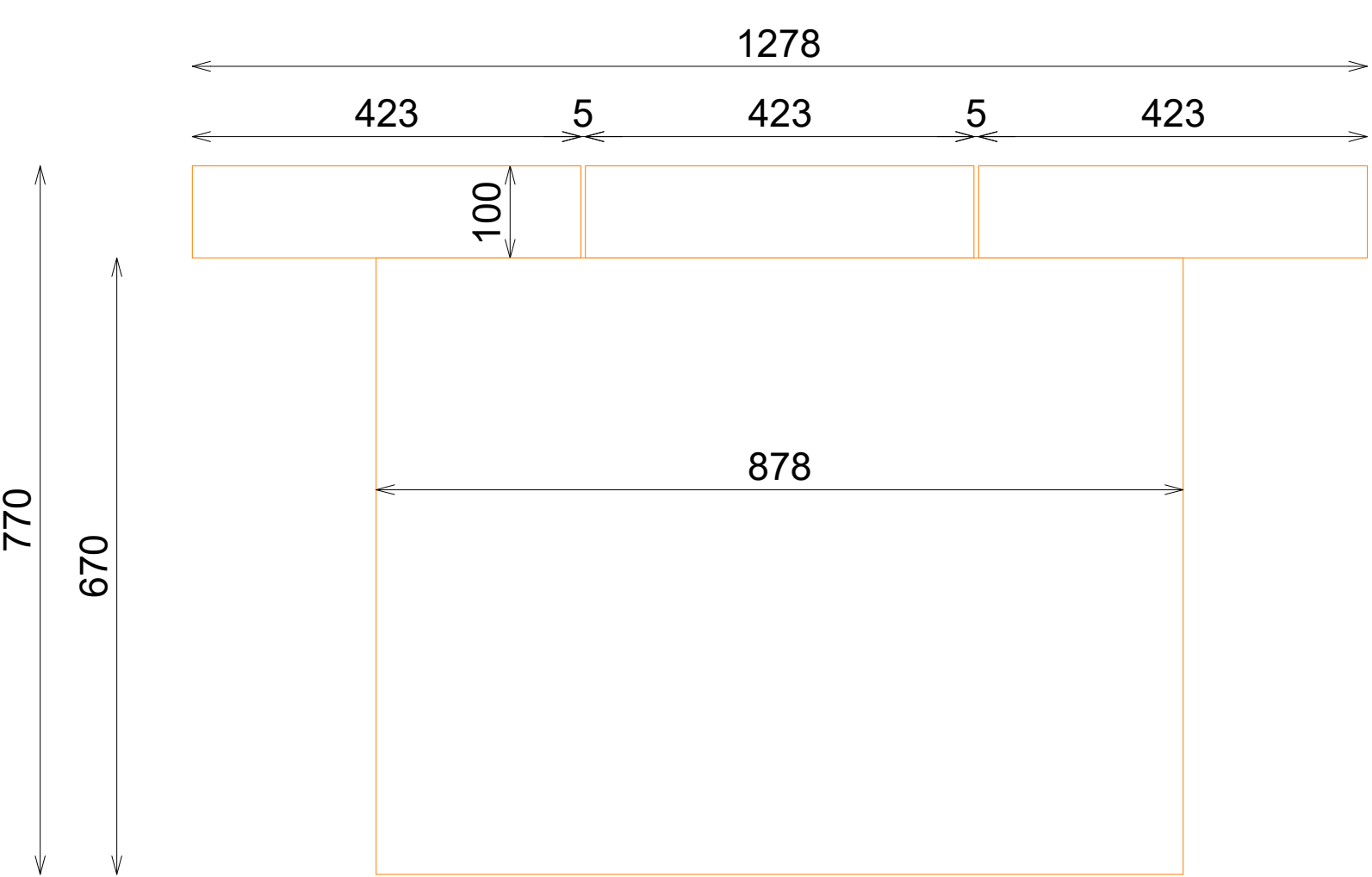
ALZADO LATERAL
