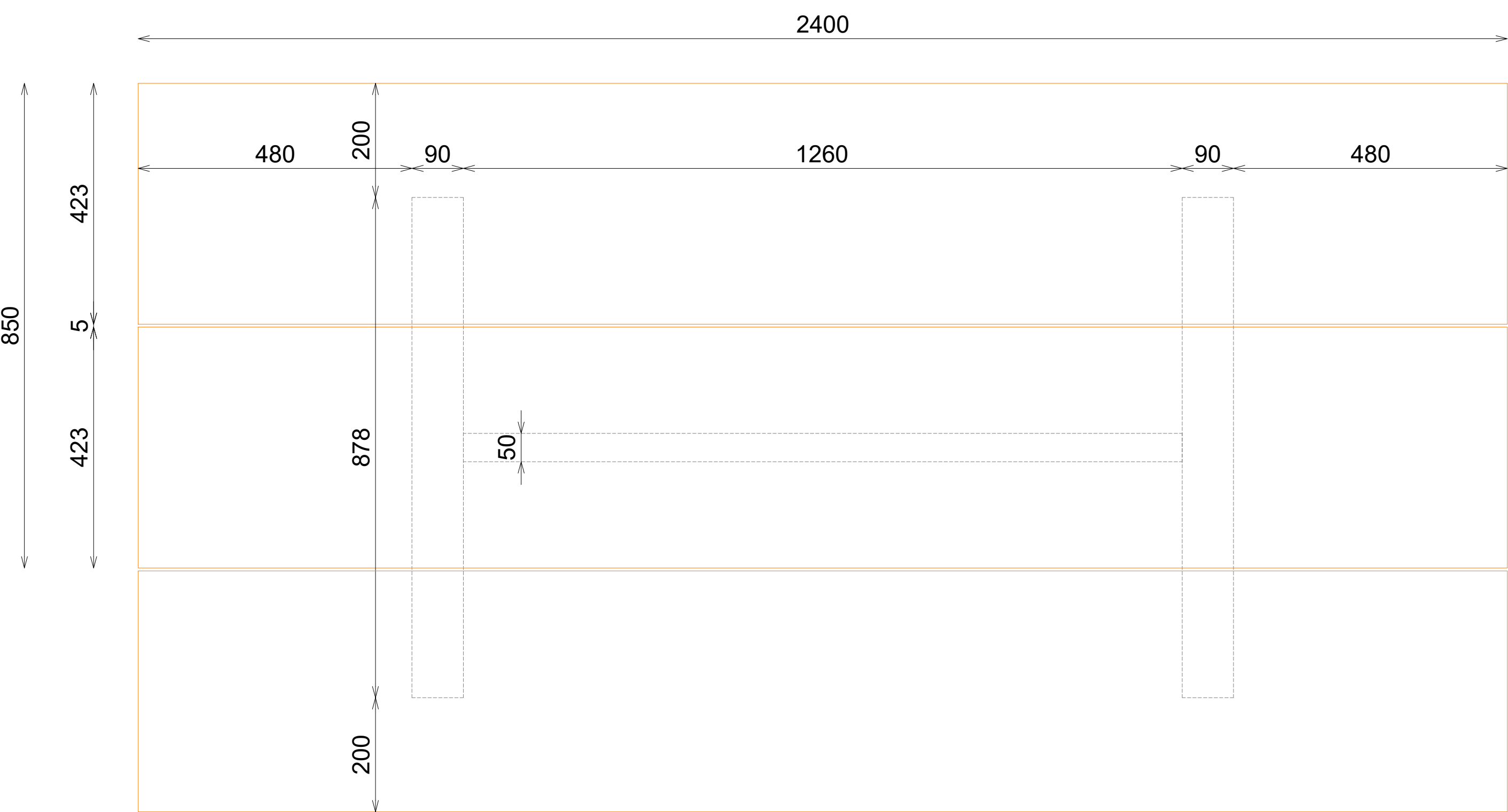
PLANTA
