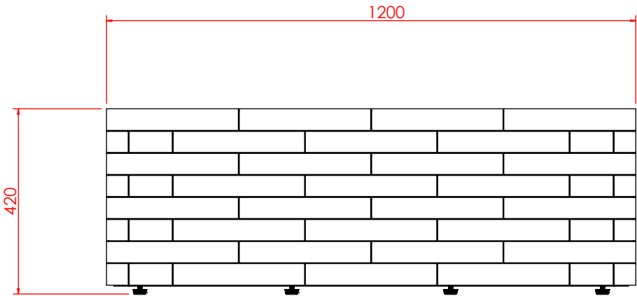
正立面
