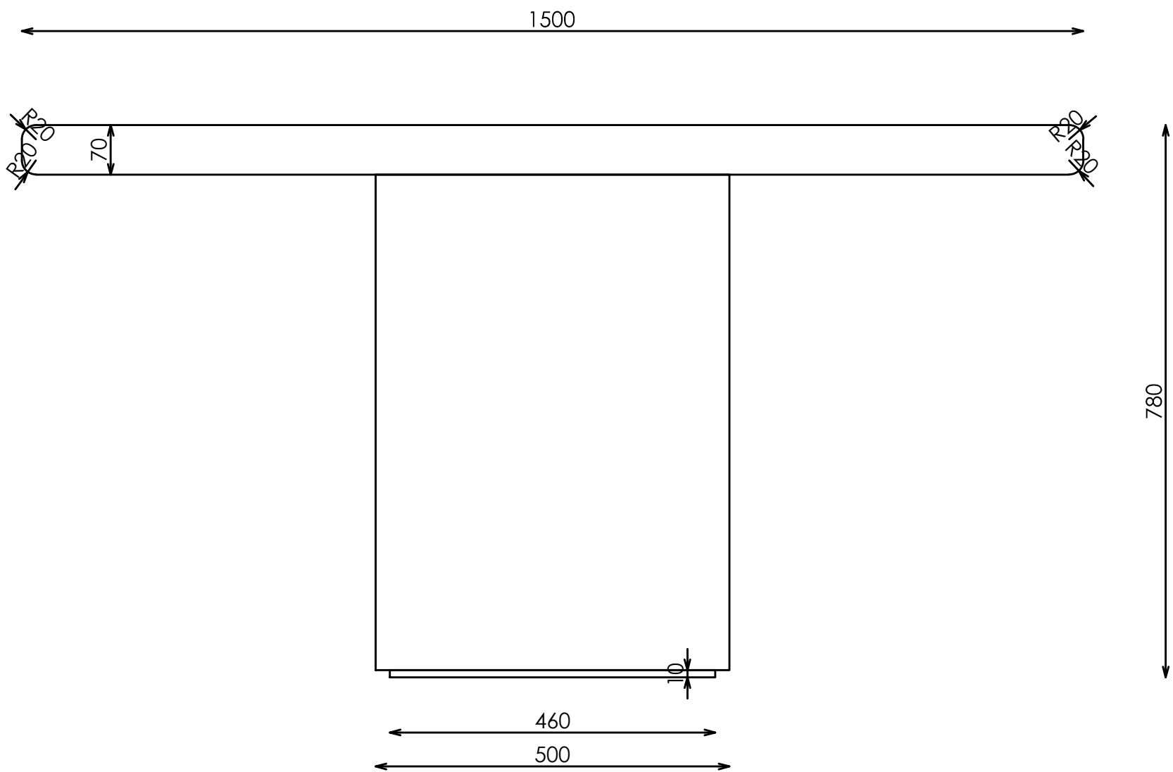
ALZADO
