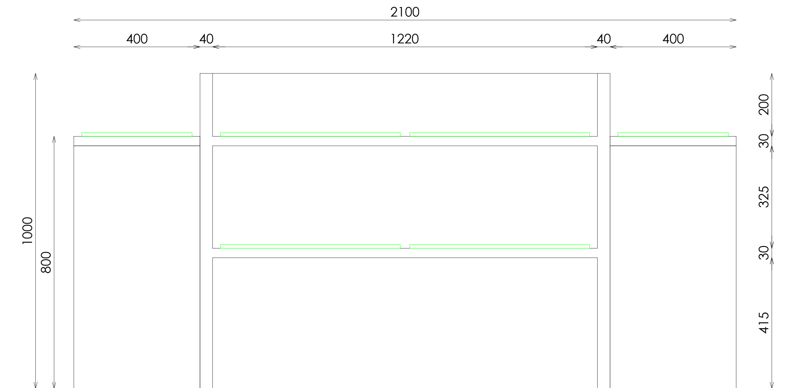
ALZADO FRONTAL
