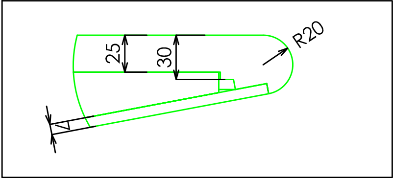
DETALLE K
