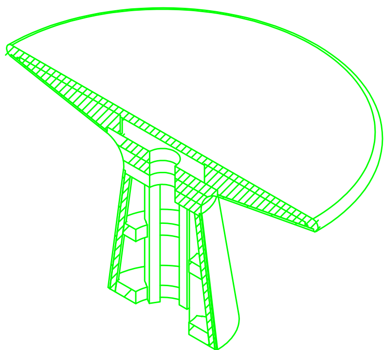
SECCIÓN ISOMETRÍA
