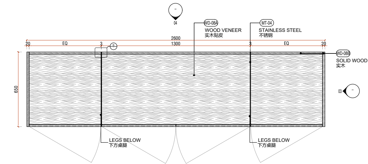
1 平面图 1:10 PLAN
