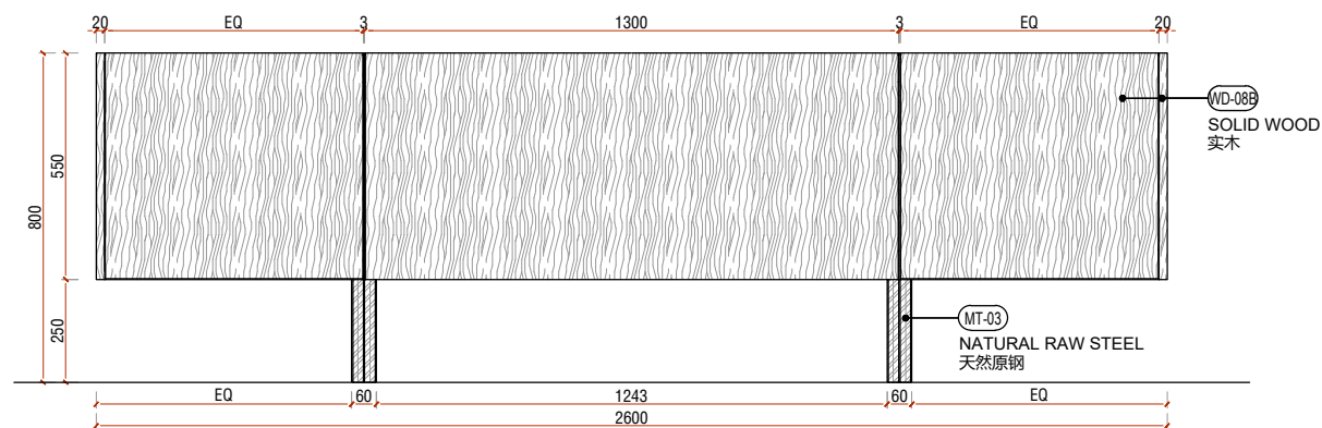
4 后立面 1:10 BACK ELEVATION
