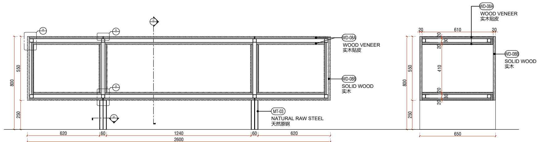
1 剖面 1:10 SECTION
