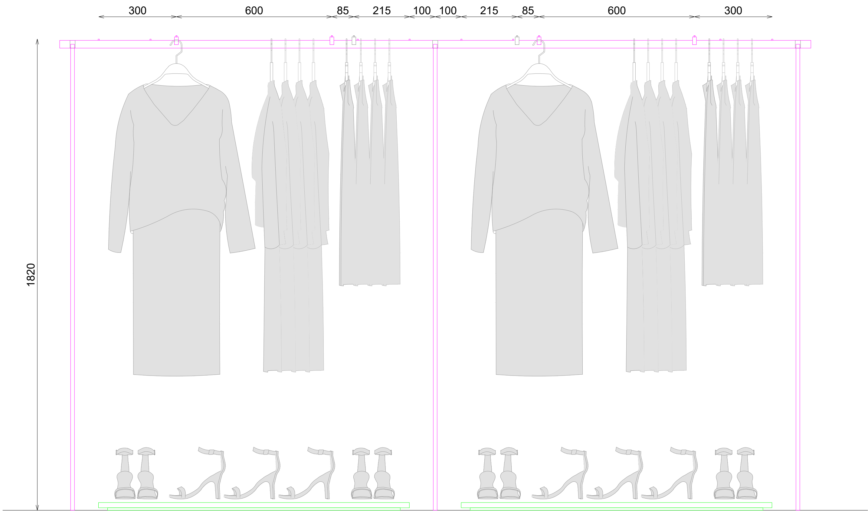
ALZADO FRONTAL
