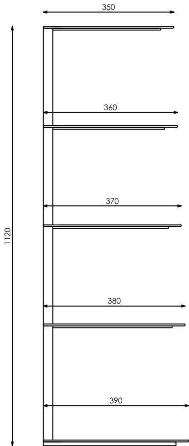
ALZADO LATERAL
