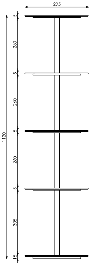
ALZADO
