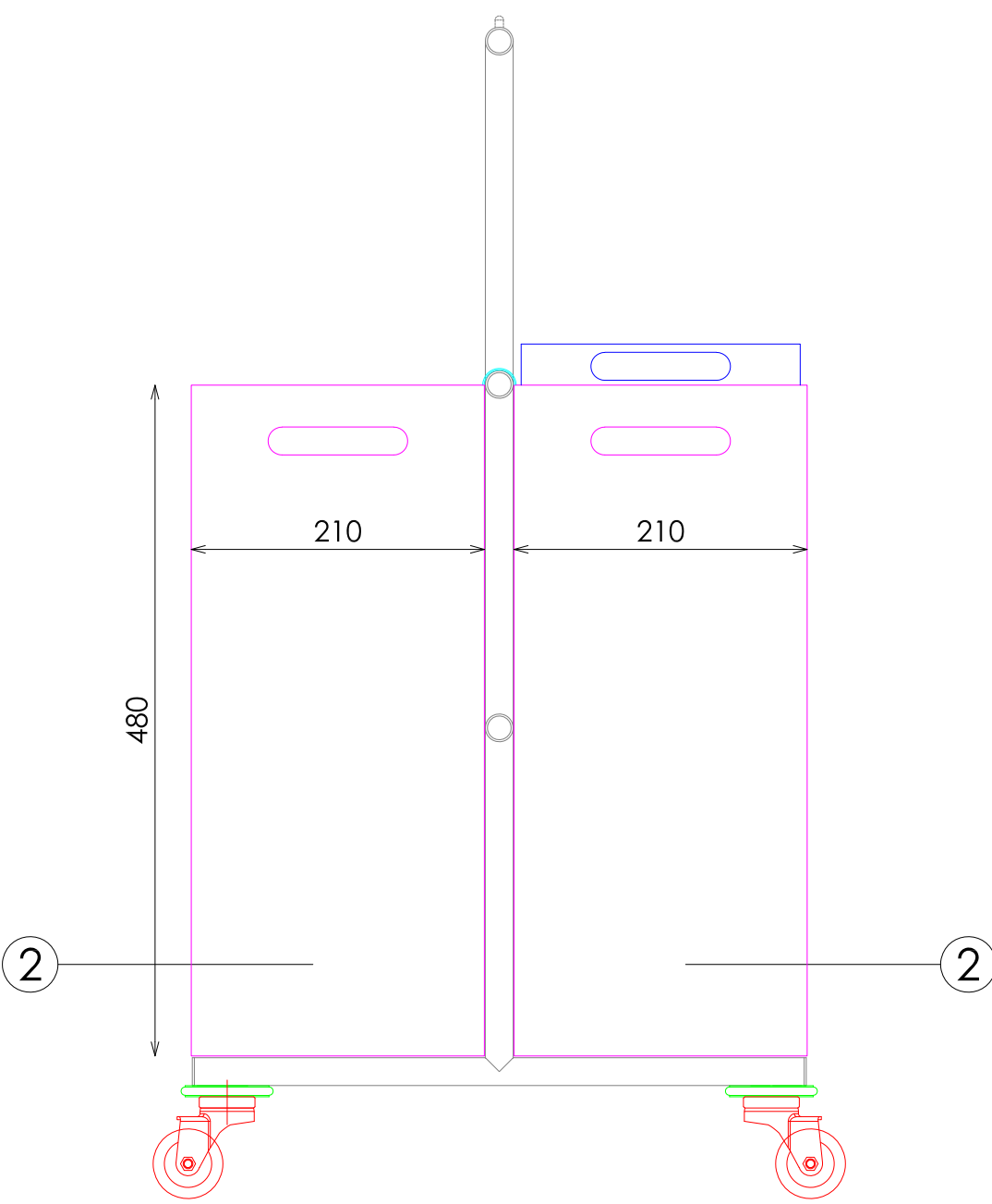
ALZADO LATERAL
