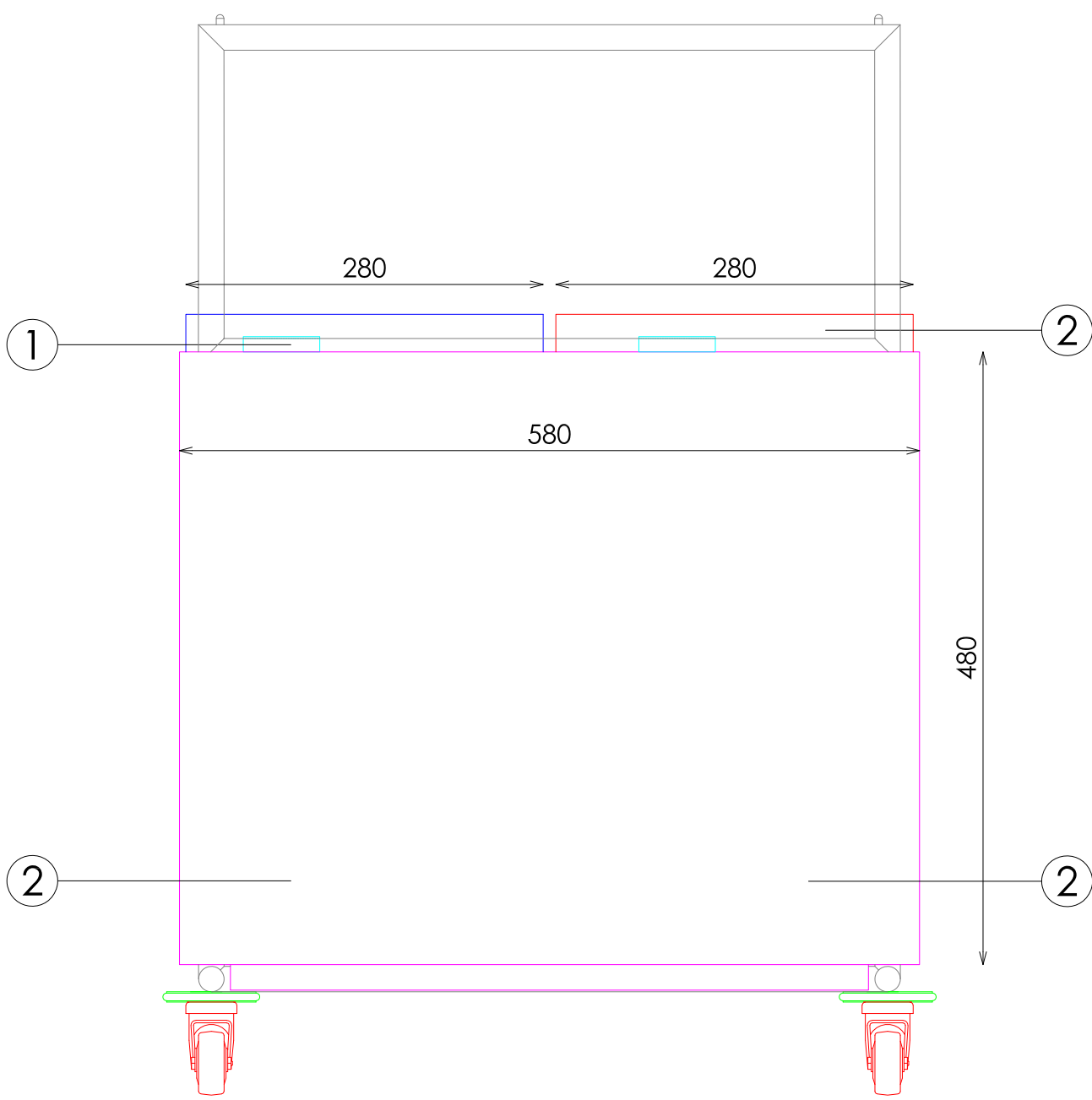
ALZADO FRONTAL
