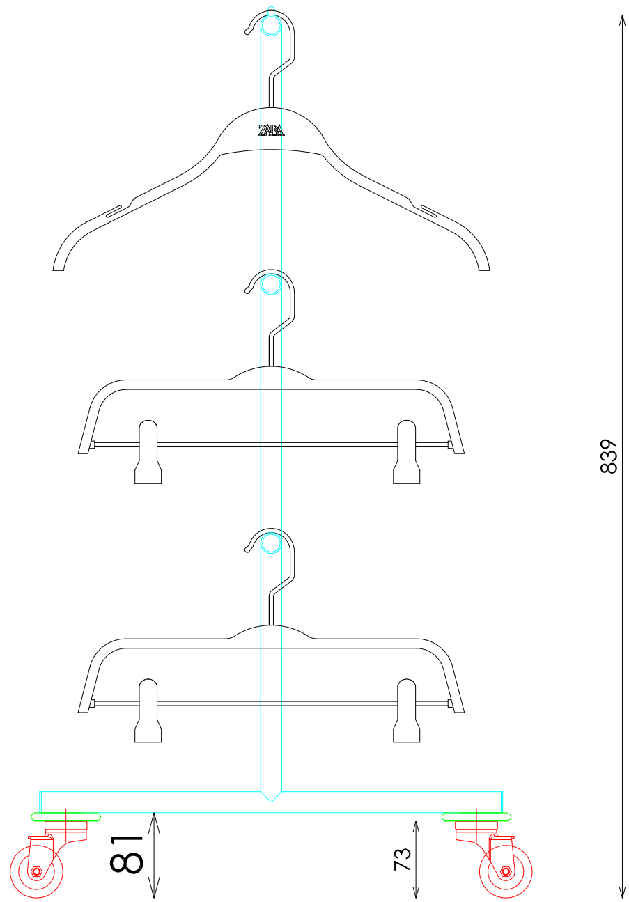
ALZADO LATERAL
