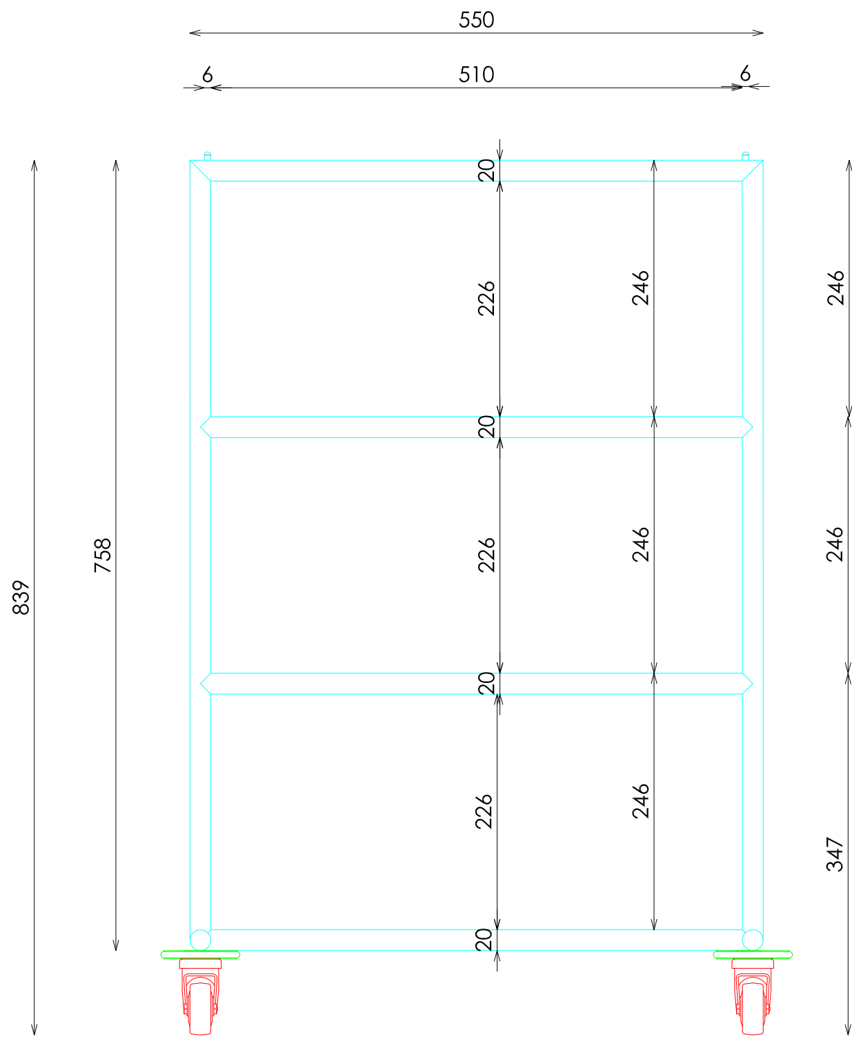
ALZADO FRONTAL
