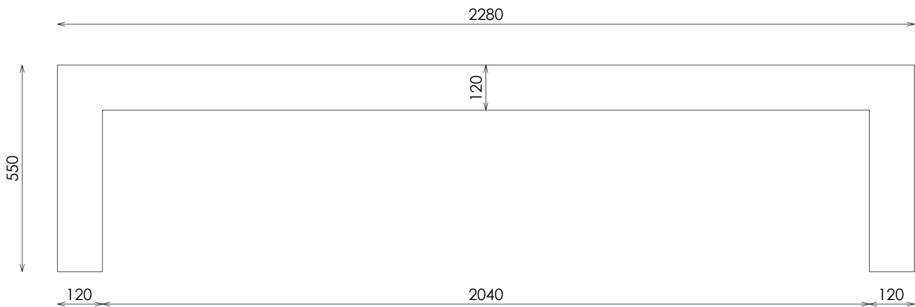
PLANTA
