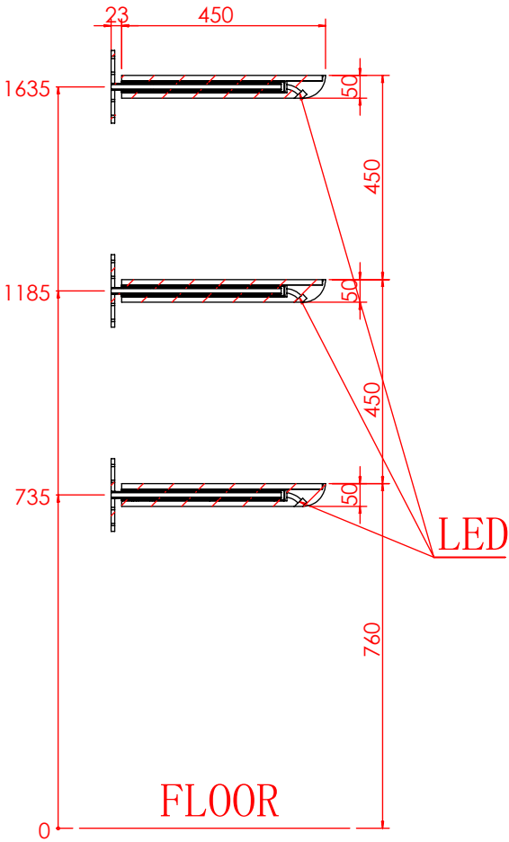
剖面 AG-AG
