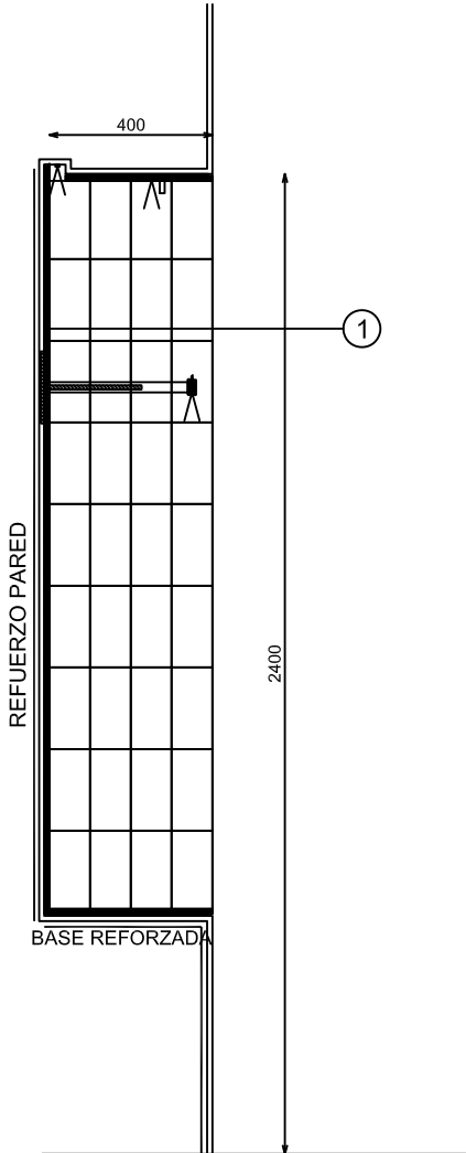
SECCION
