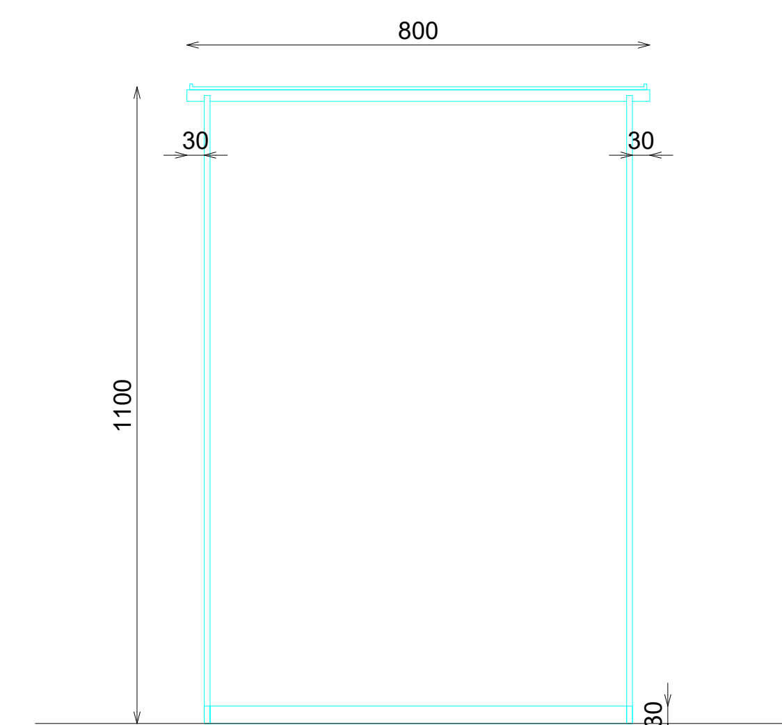
ALZADO
