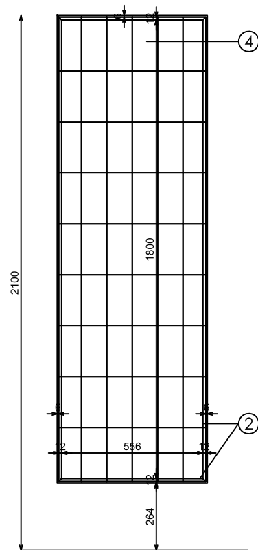
ALZADO
