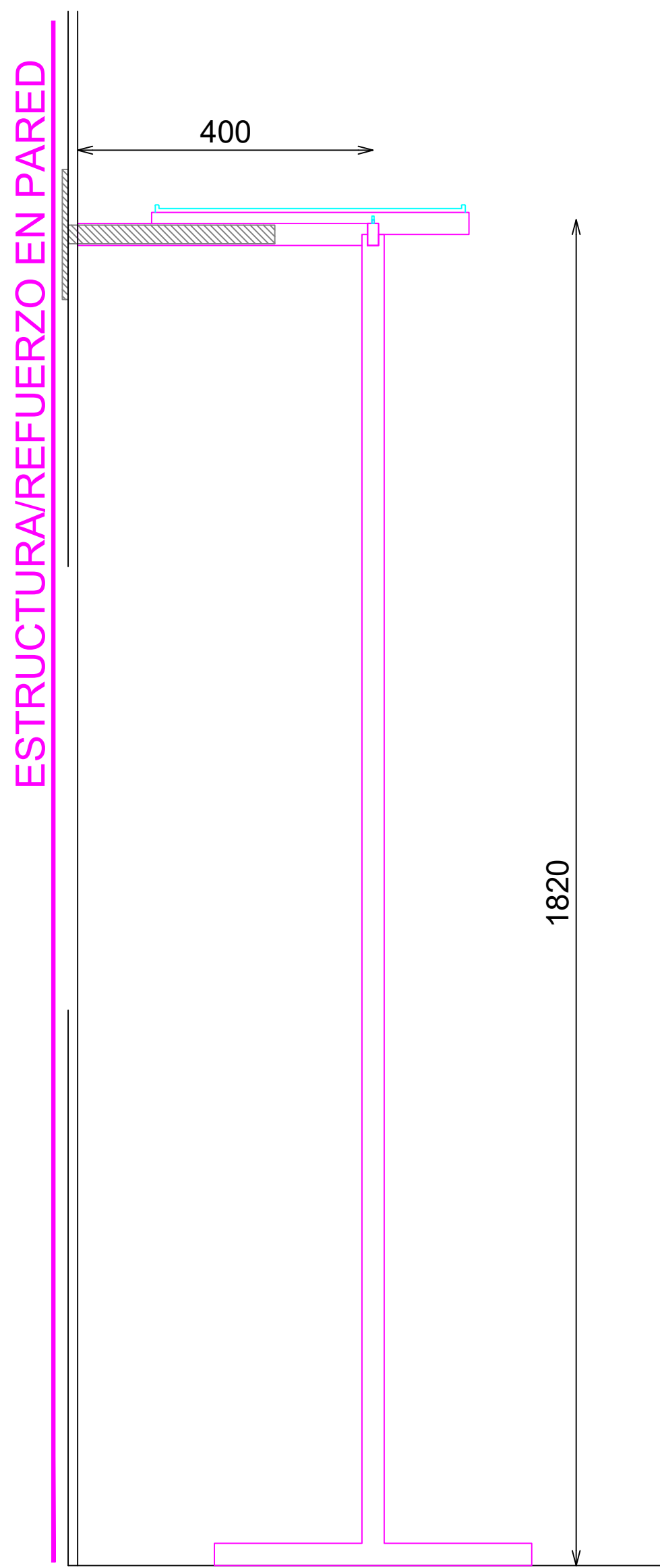
SECCION
