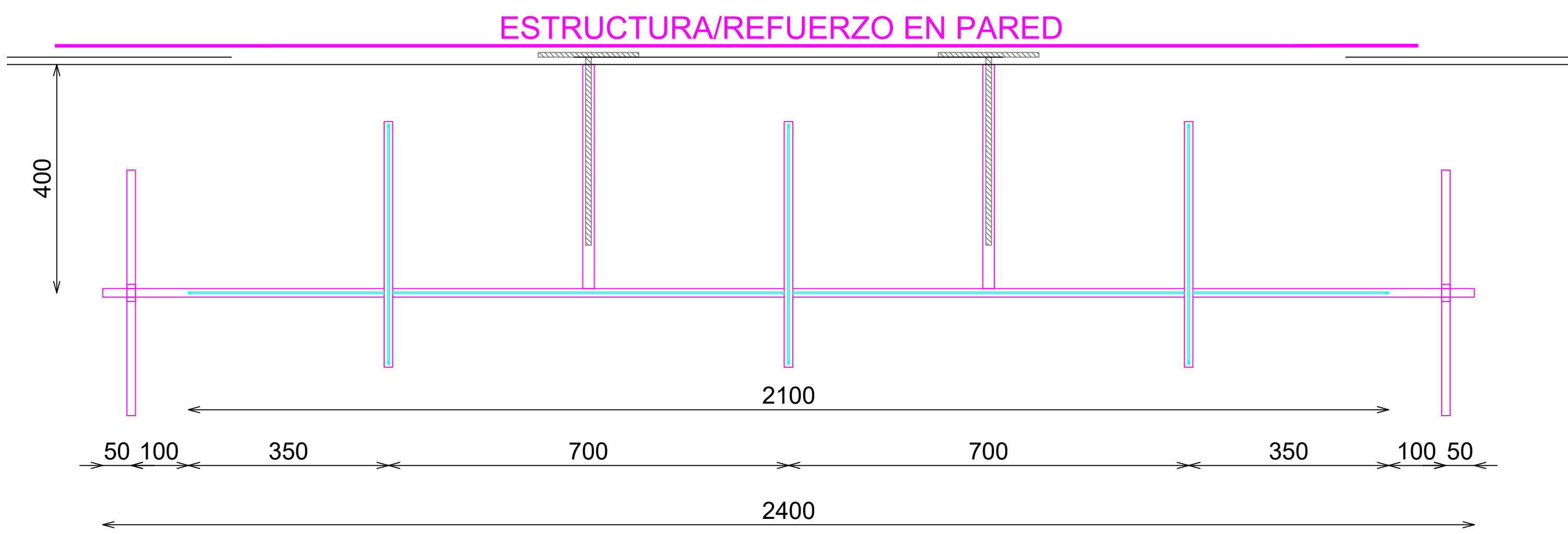
PLANTA
