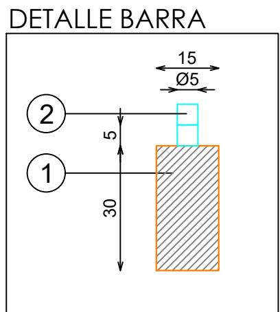
DETALLE BARRA
