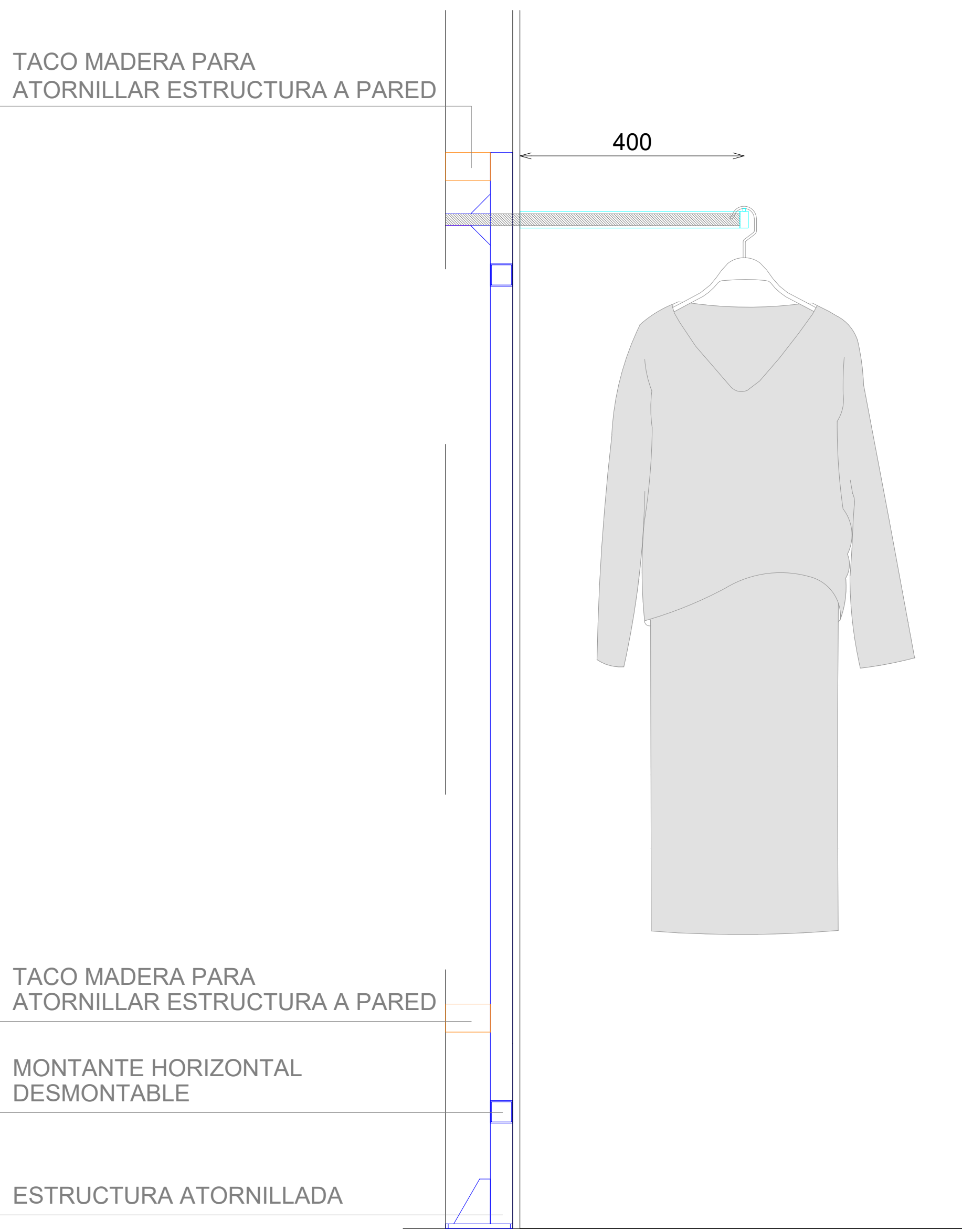
SECCION
