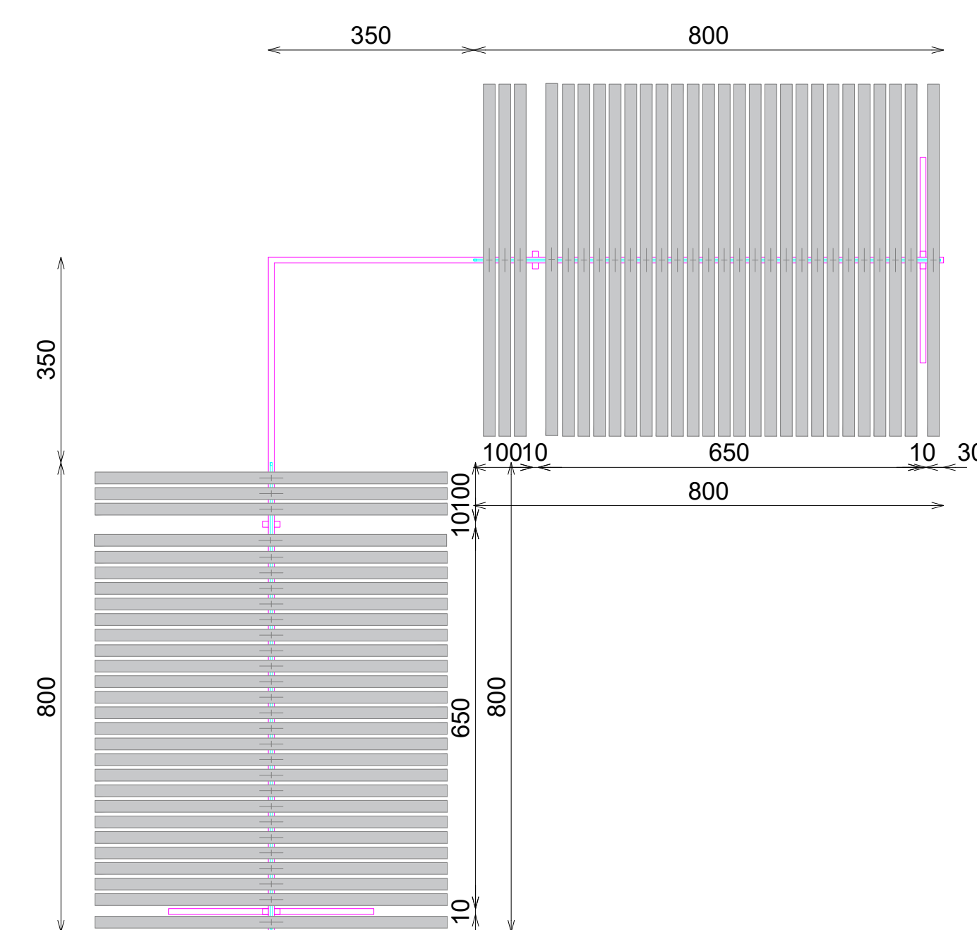
PLANTA
