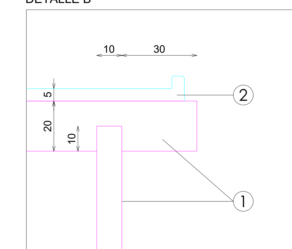
DETALLE B
