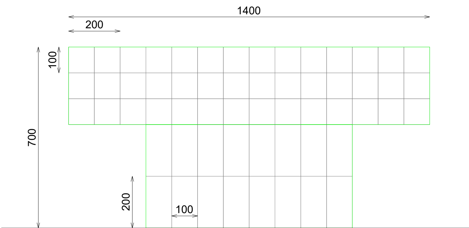
PERFIL
