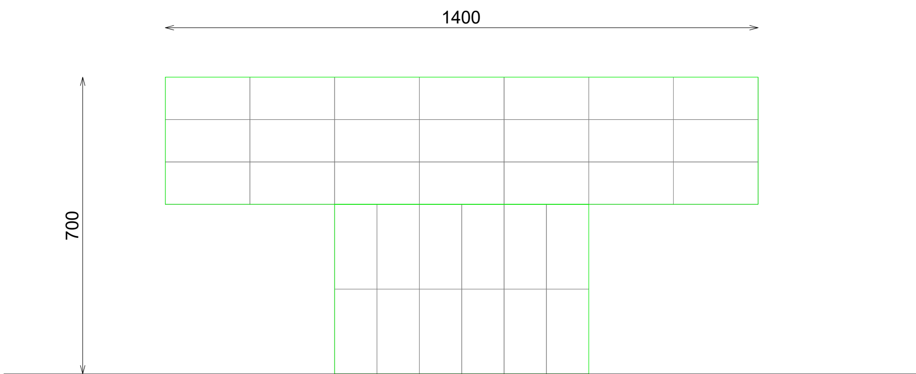
ALZADO
