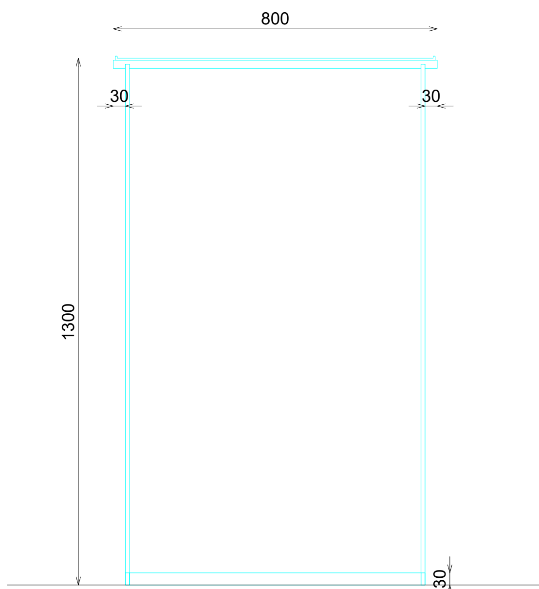
ALZADO
