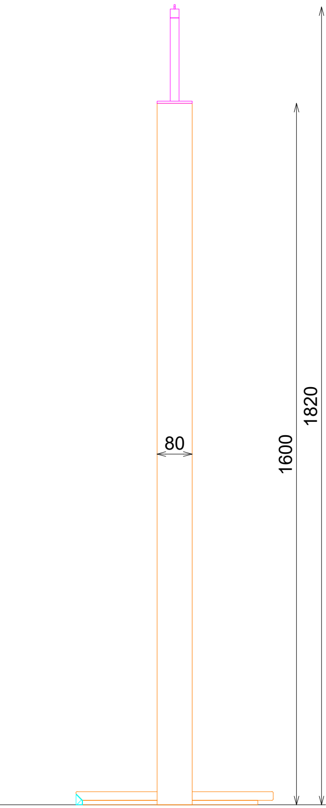
PERFIL
