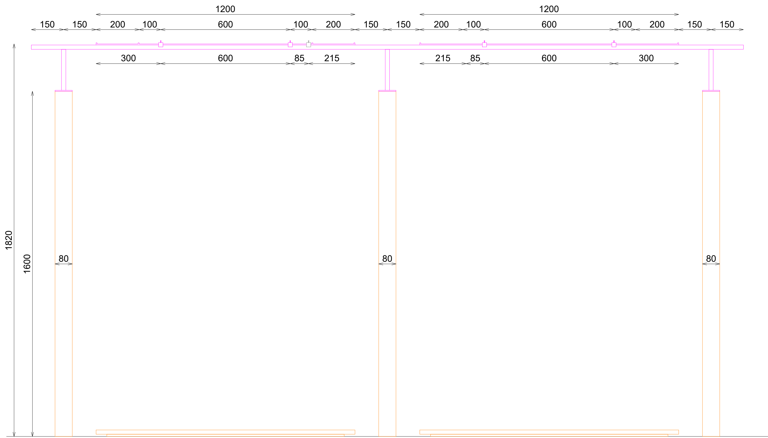
ALZADO FRONTAL
